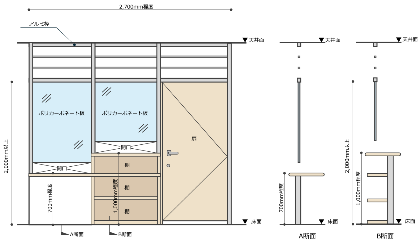
窓口カウンター 参考イメージ図（事務室①側姿図）
