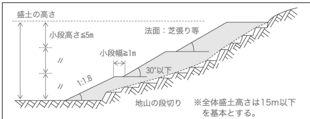
図：盛土のり面の形状
