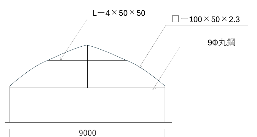
通り軸組図
