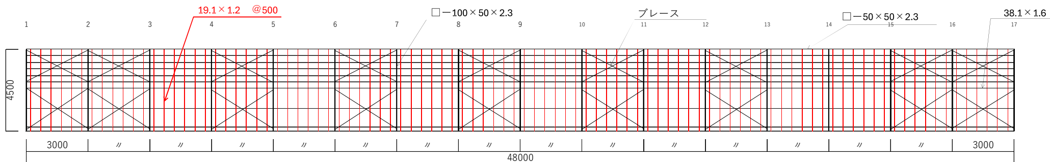
通り姿図
