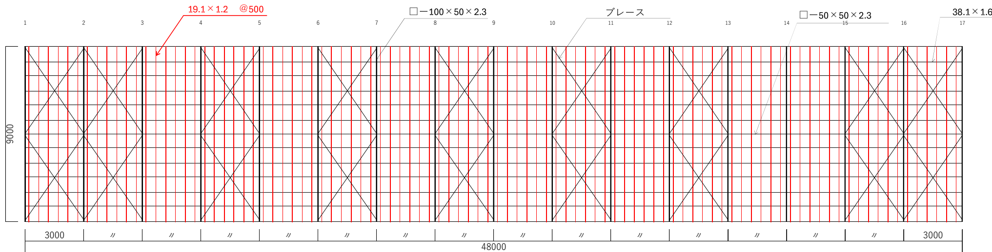
小屋伏図
