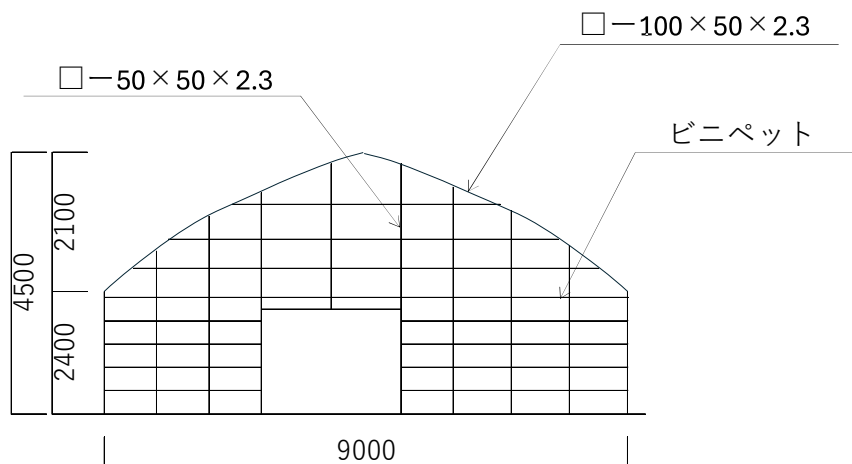
正面図
