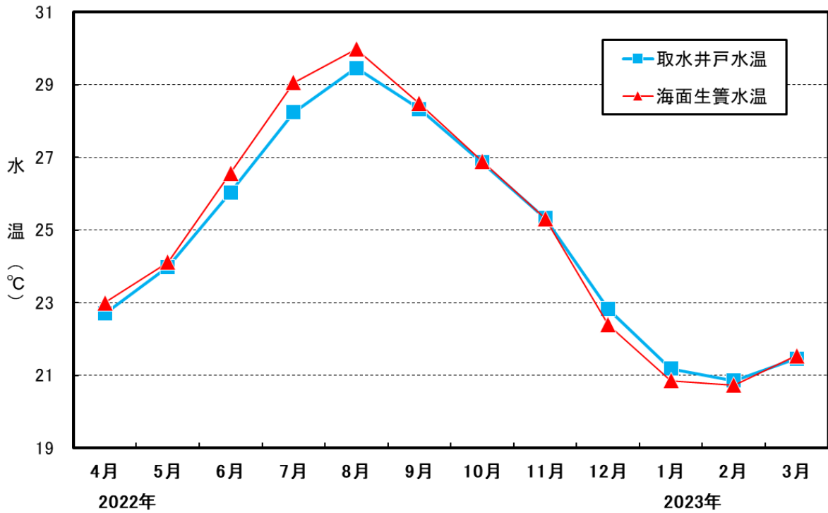
資料4 2022年の取水井戸及び海面生簀の月平均水温の推移
