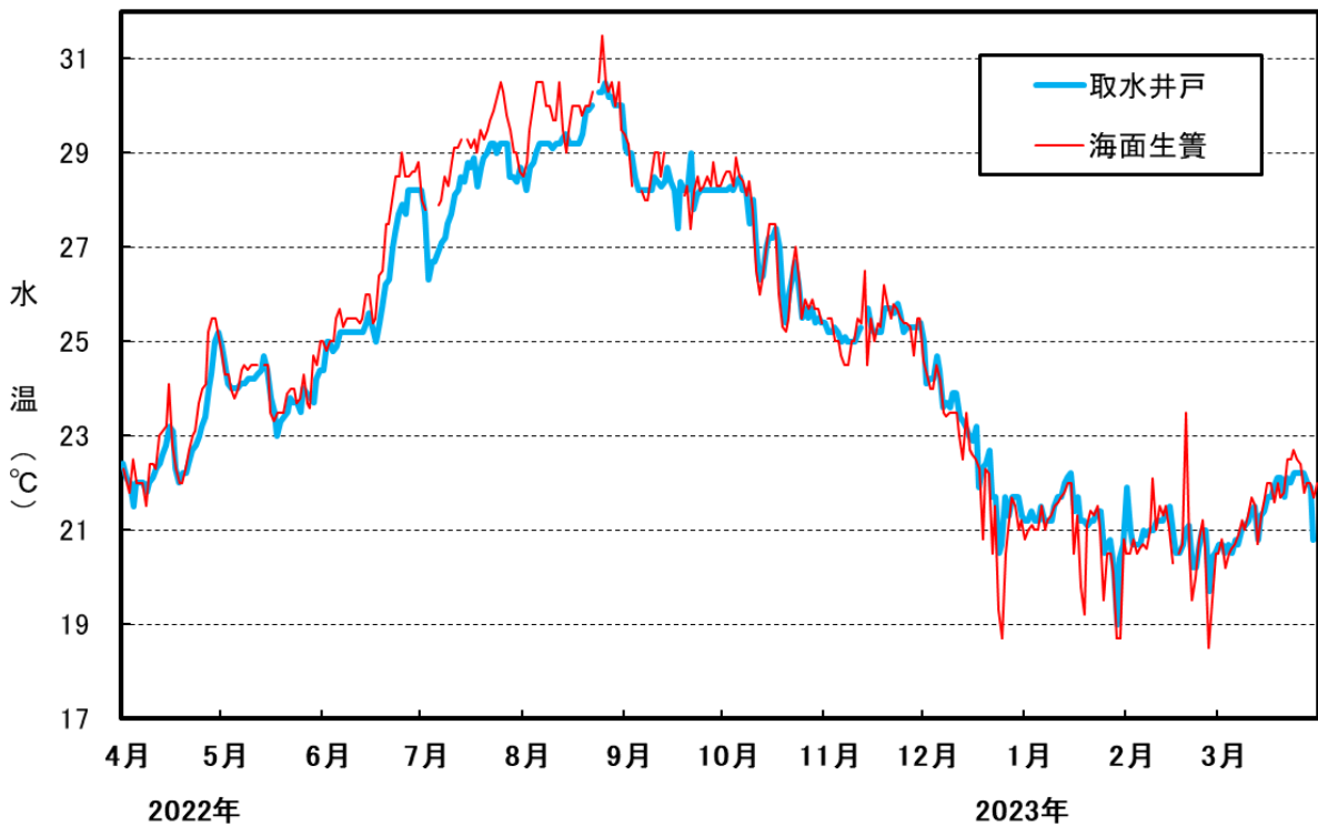
資料5 2022年の取水井戸及び海面生簀の日毎水温の推移
