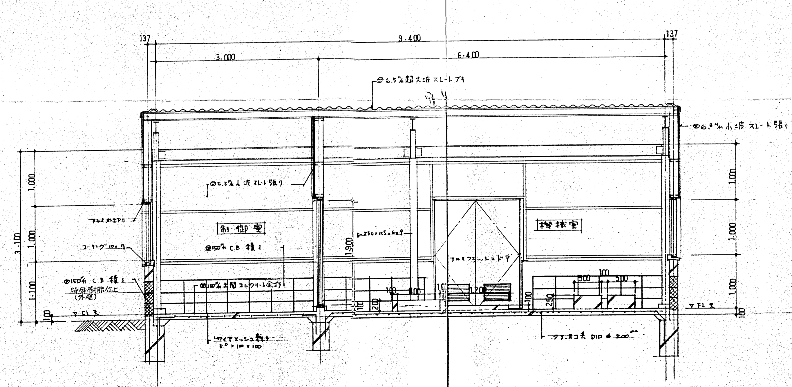
2 断面詳細図 1:40
