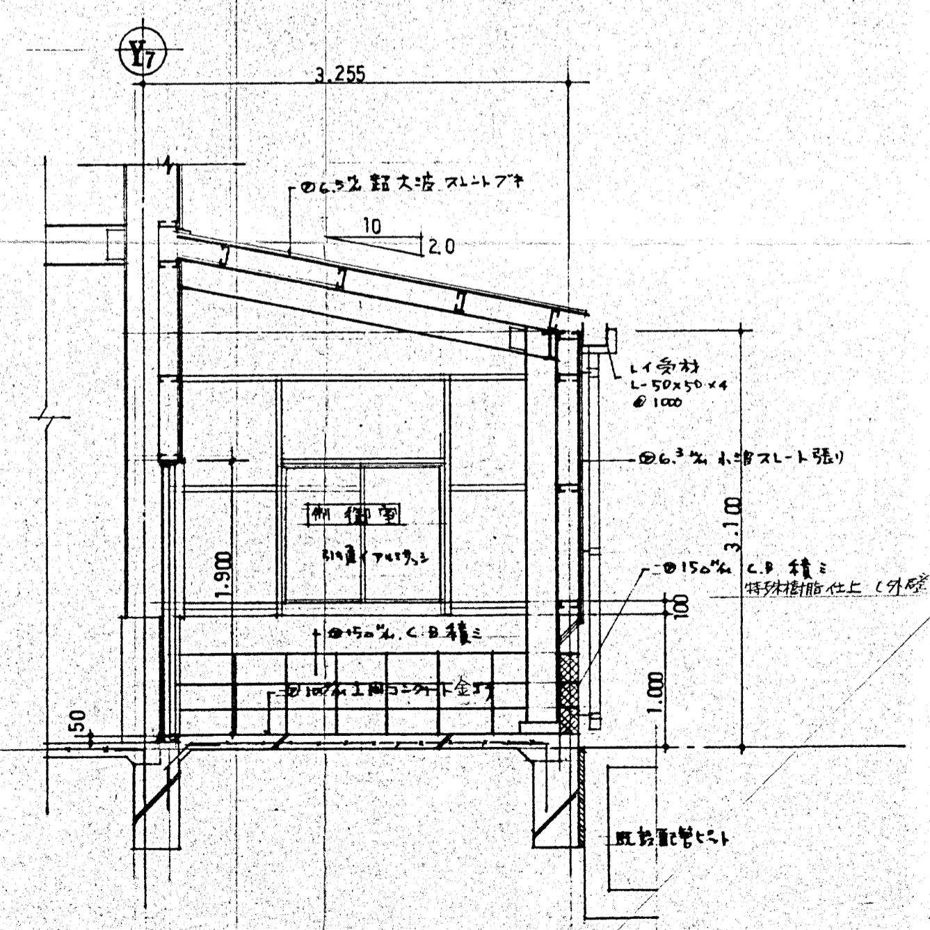
3 断面詳細図 1:40
