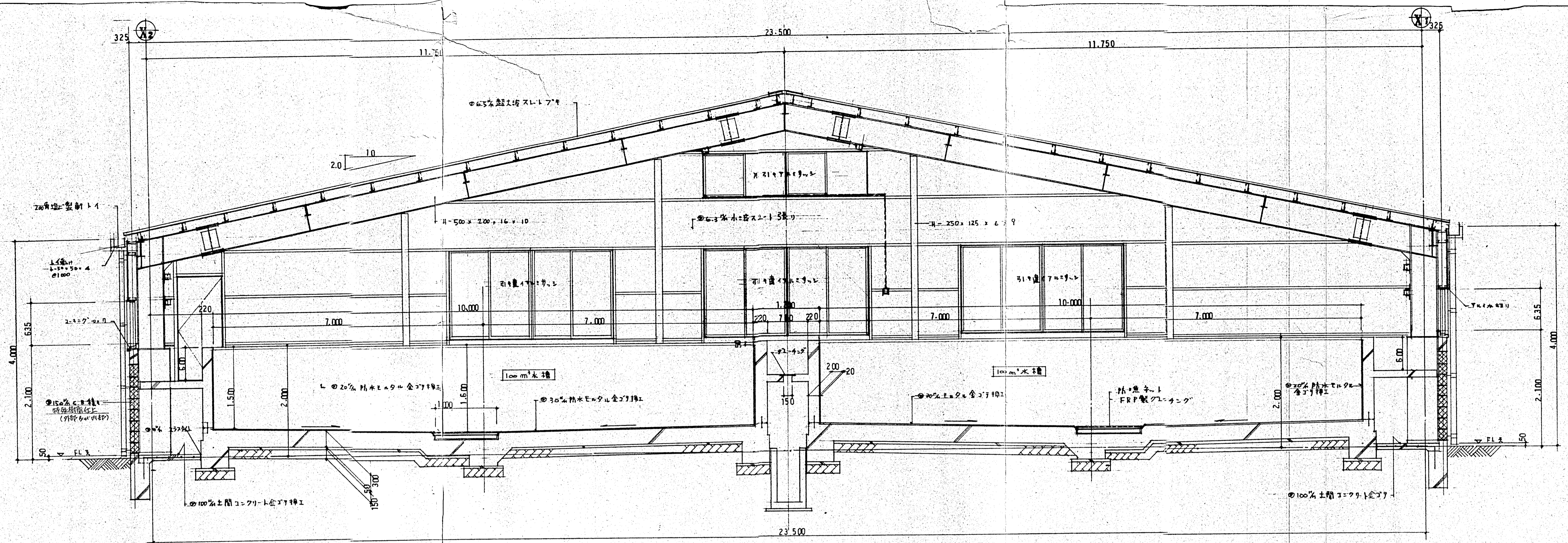
1 断面詳細図 1:40
