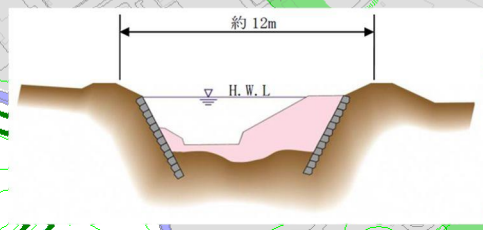
標準断面図
