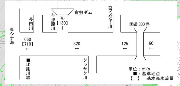
計画高水流量配分図
