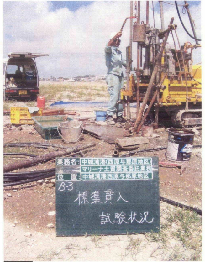
B-3 標準貫入試験
