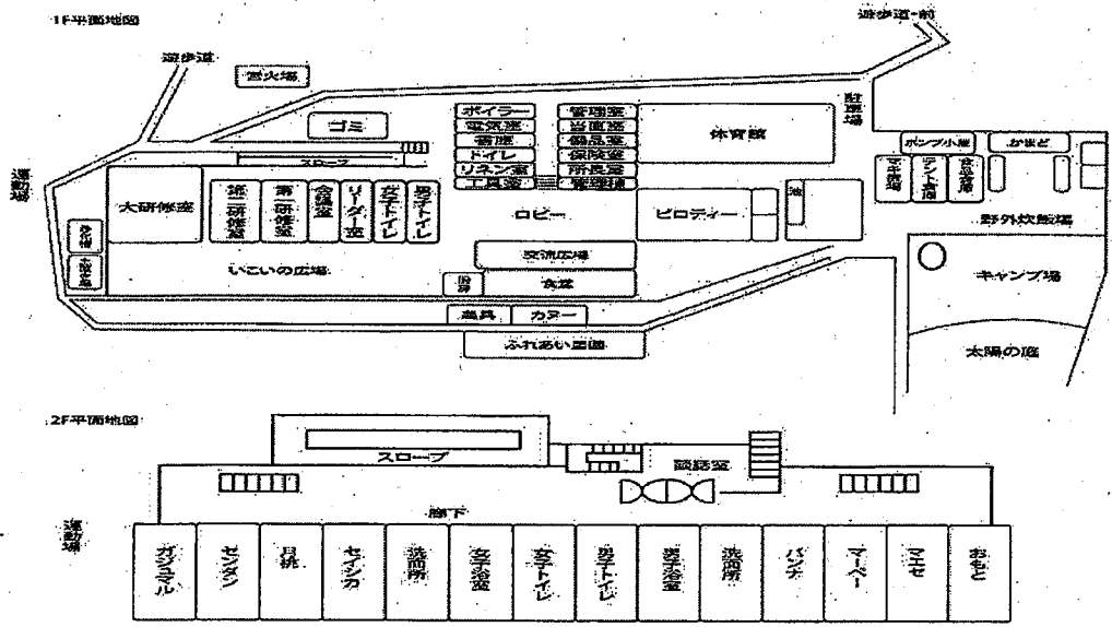
沖縄県立石垣青少年の家 配置図
