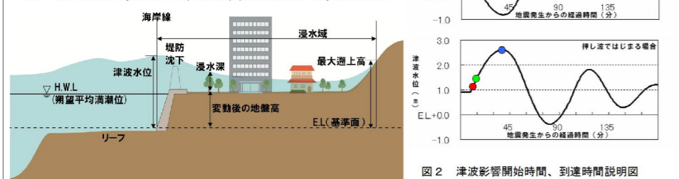
図2 津波影響開始時間、到達時間説明図
