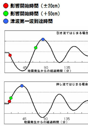
図2 津波影響開始時間、到達時間説明図
