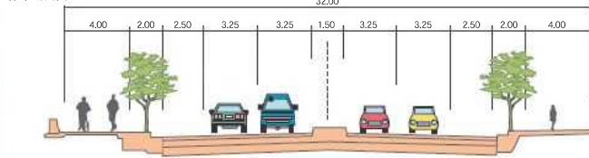
標準断面図
