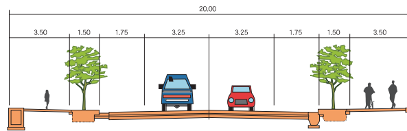
標準断面図
