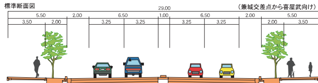
標準断面図
