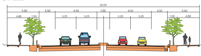
標準断面図
