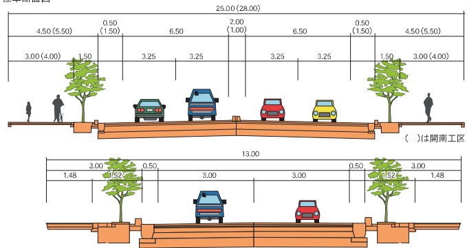
標準断面図
