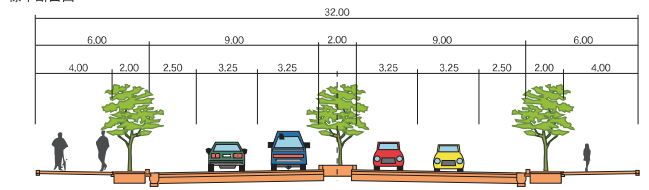
標準断面図
