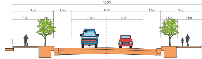
標準断面図
