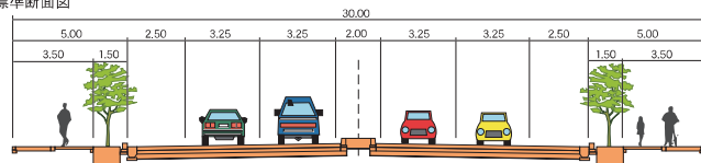
標準断面図
