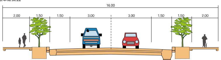
標準断面図
