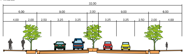
標準断面図
