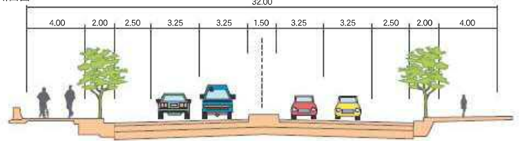
標準断面図
