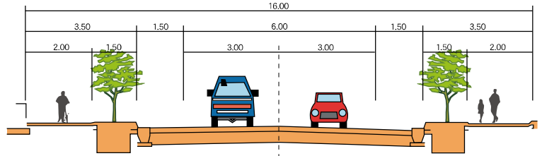
標準断面図
