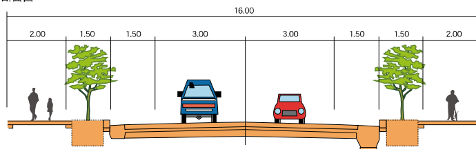
標準断面図
