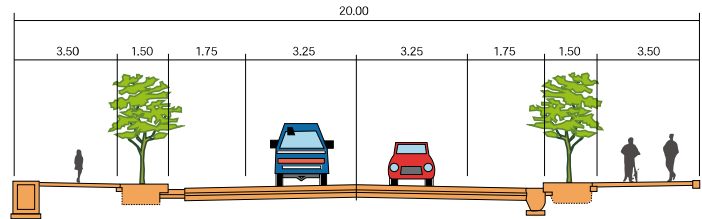
標準断面図
