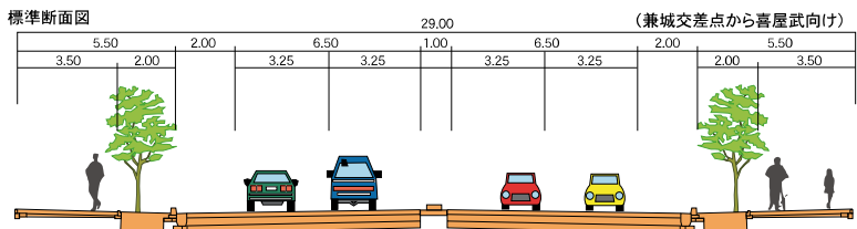
標準断面図
