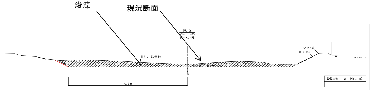
標準断面図
