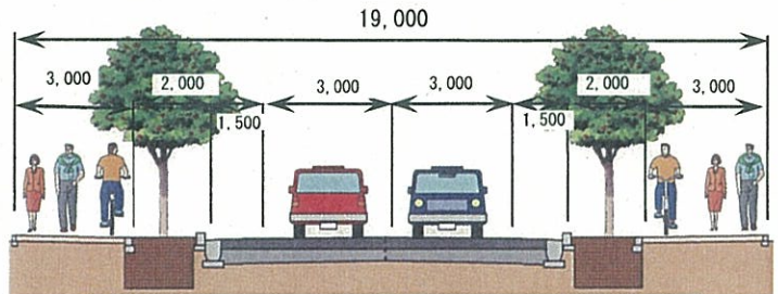
真壁集落 (W=19.0m、今回計画)
