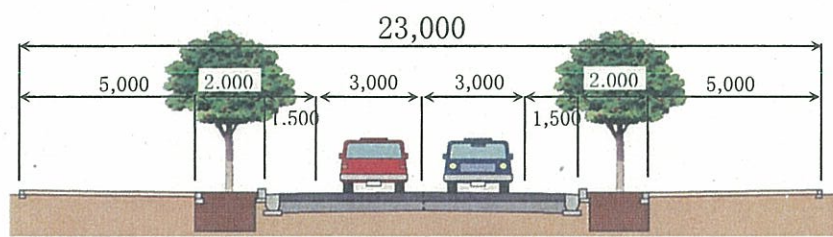
国吉～米須 (W=23.0m、H16再評価時点)
