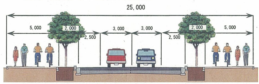
照屋～国吉 (W=25.0m、施工済箇所)
