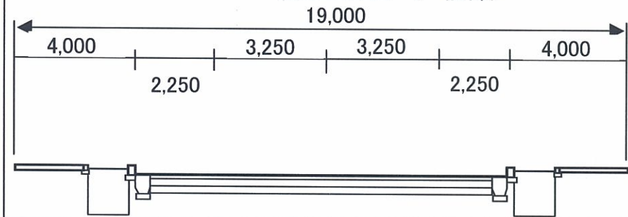
標準断面 (一般部)
