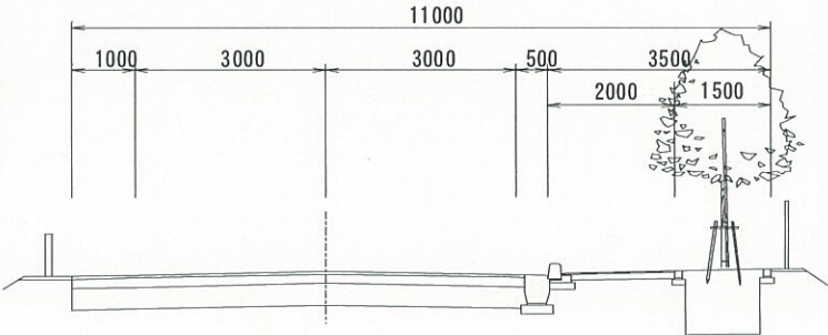
標準断面
