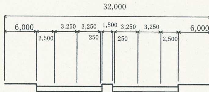
標準断面図
