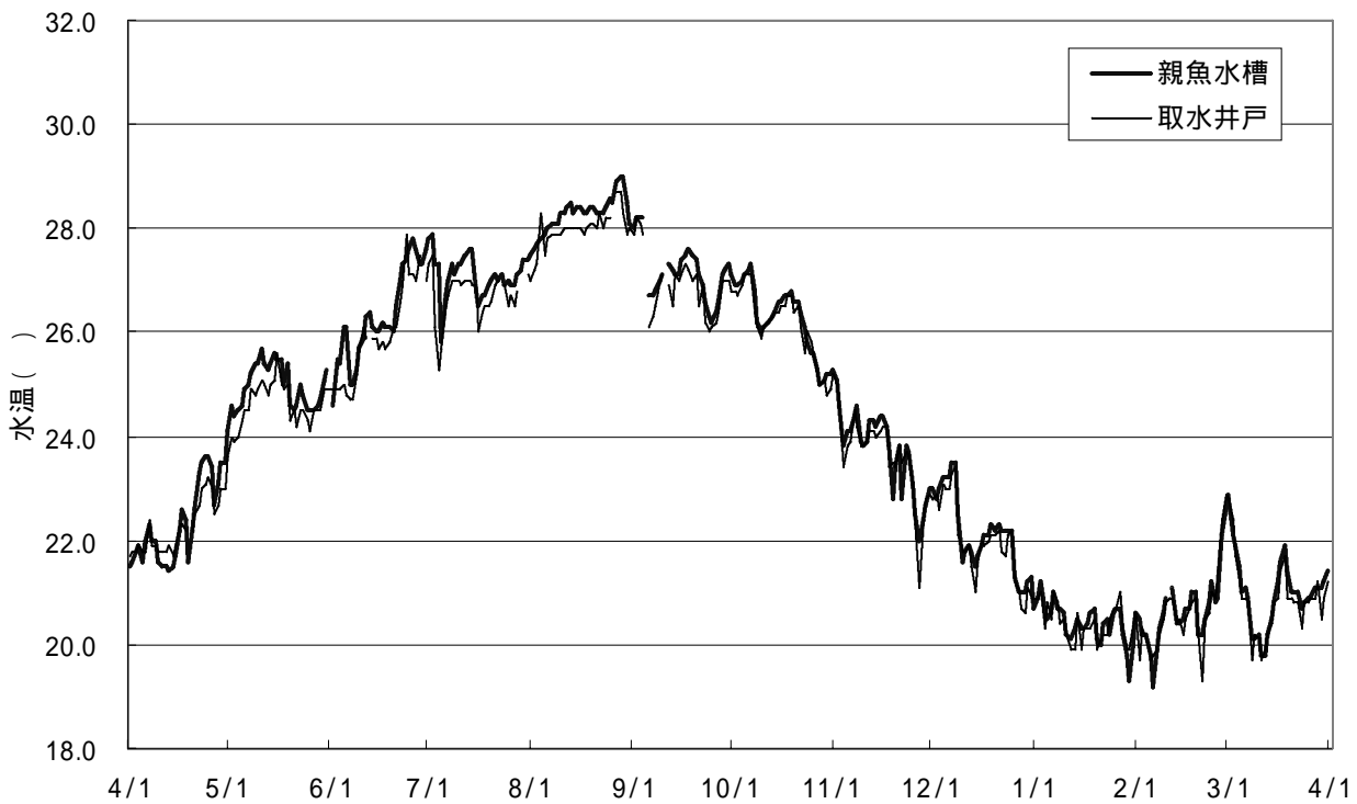
図1 平成14年(2002年)栽培漁業センター親魚水槽及び取水井戸水温の推移
