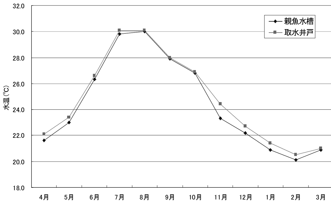
図2 平成13年(2001年)親魚水槽及び取水井戸平均水温の推移
