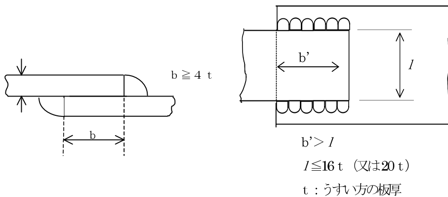
図 11-2-2 前面すみ肉溶接の重ね代 (b) 図 11-2-3 側面すみ肉溶接の重ね代 (b')
