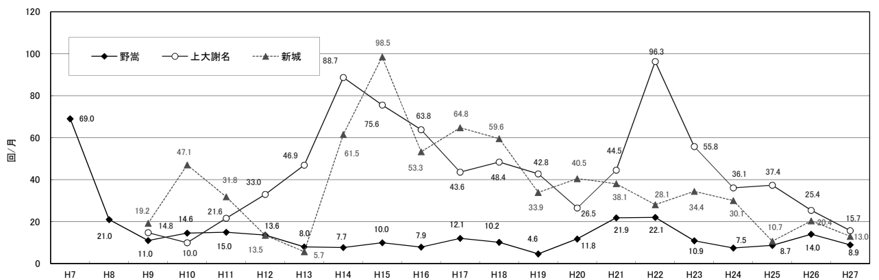
図F10-2 航空機騒音規制措置合意前後の航空機騒音発生状況 (騒音発生回数の年度別推移、夜間(22時)～早期(7時))
