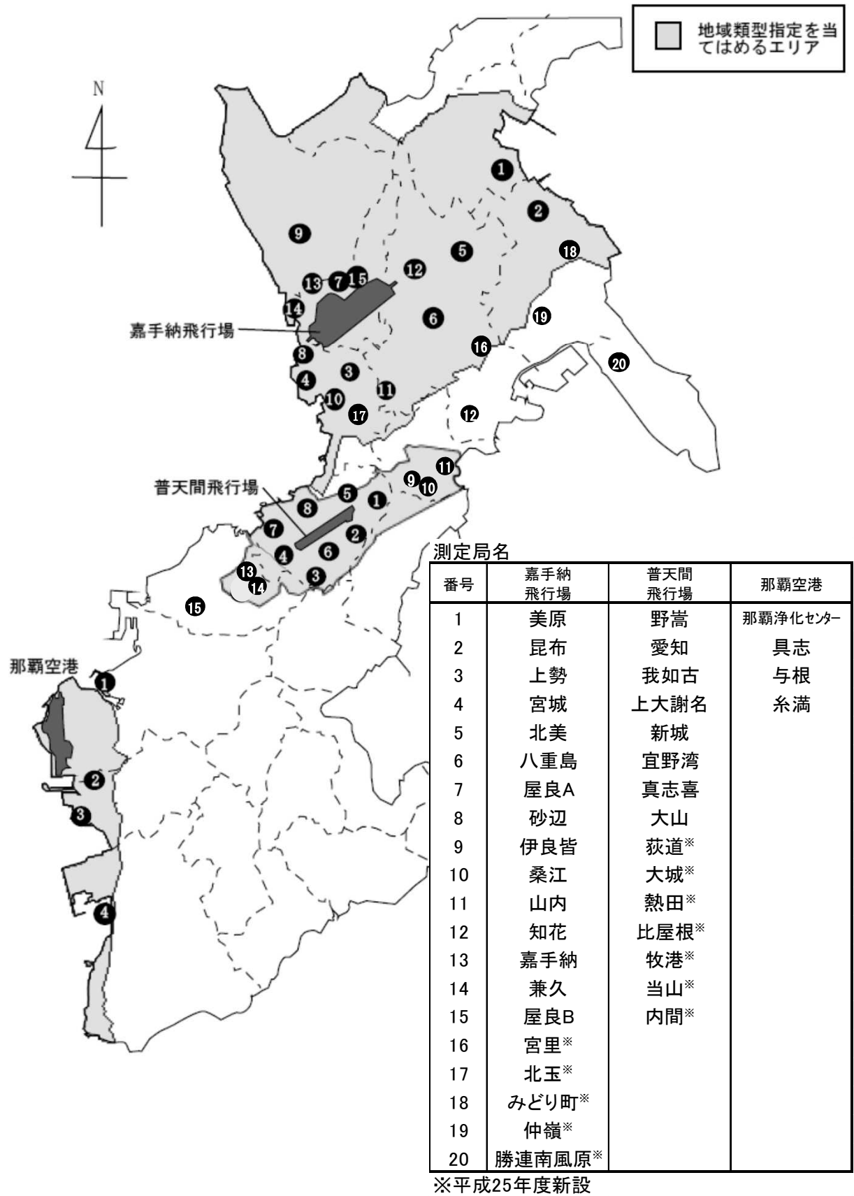
図1 航空機騒音測定局配置図
