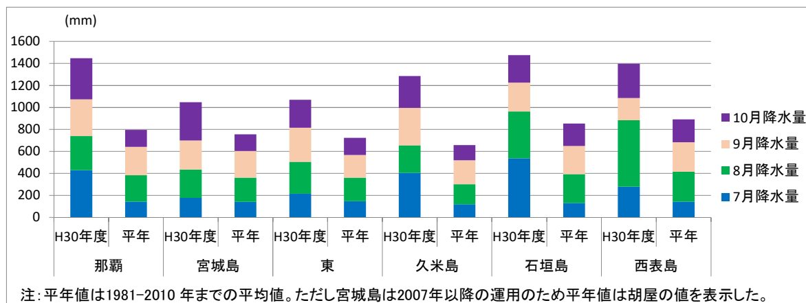
図 2.2-3 H30年7-10月(夏季から初秋)の総降水量の比較
