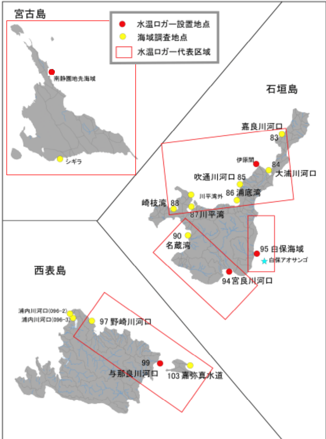
図 2.3-2 ロガー設置位置図 (2/2)
