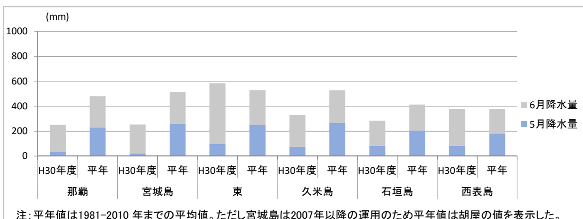
図 2.2-2 H30年5-6月(梅雨時)の総降水量
