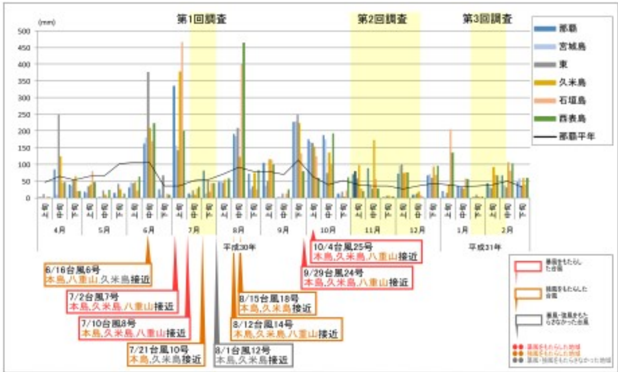
図 2.2-1 今年度(H30年度)の旬別降水量及び台風接近時期
