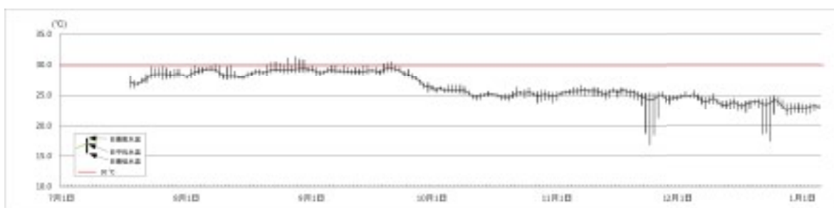
図 2.3-3 大小堀川河口 022-2 海水温データ
