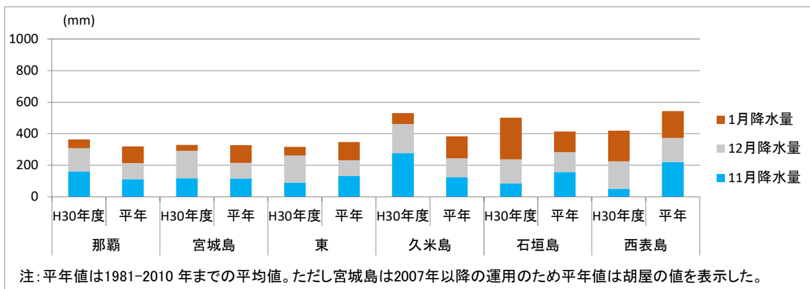
図 2.2-4 H30年11月-H31年1月(秋季から冬季)の総降水量の比較
