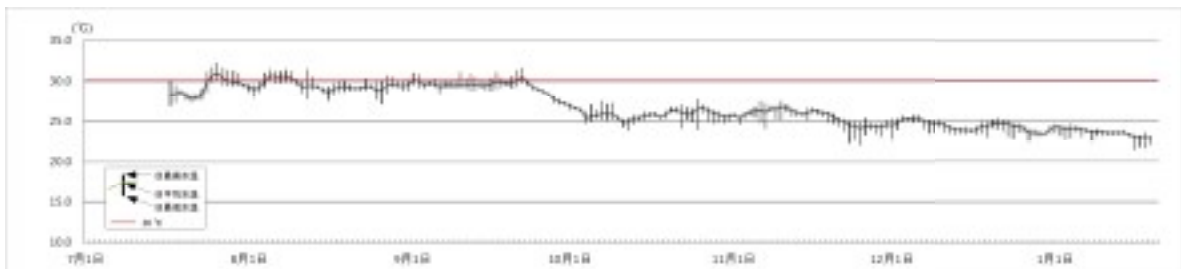
図 2.3-6 真謝川河口 071-1 における海水温データ
