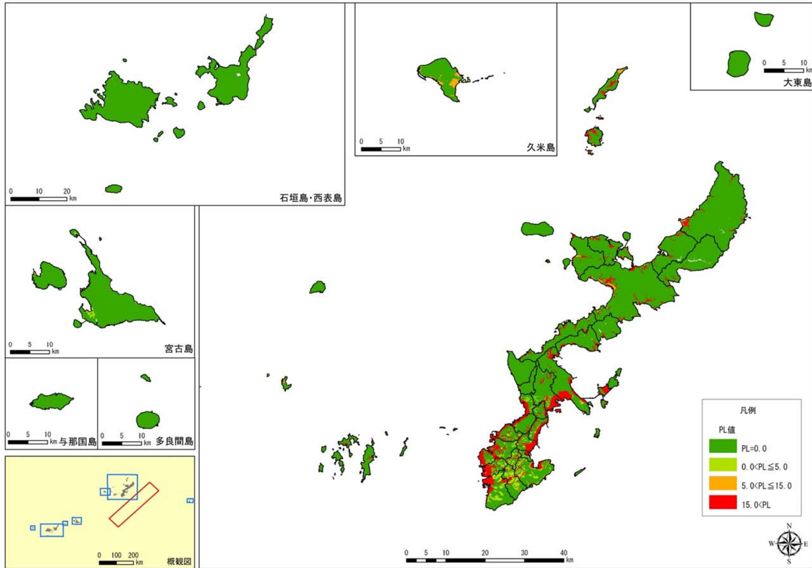
図 2.2-2(10) 沖縄本島南東沖地震の液状化危険度(PL 値)分布
