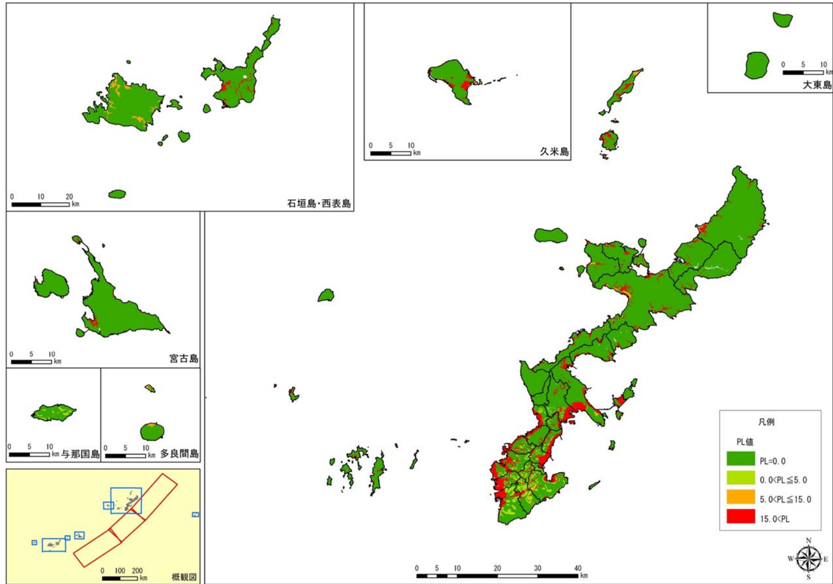
図 2.2-2(20) 沖縄本島南東沖地震3連動の液状化危険度(PL値)分布
