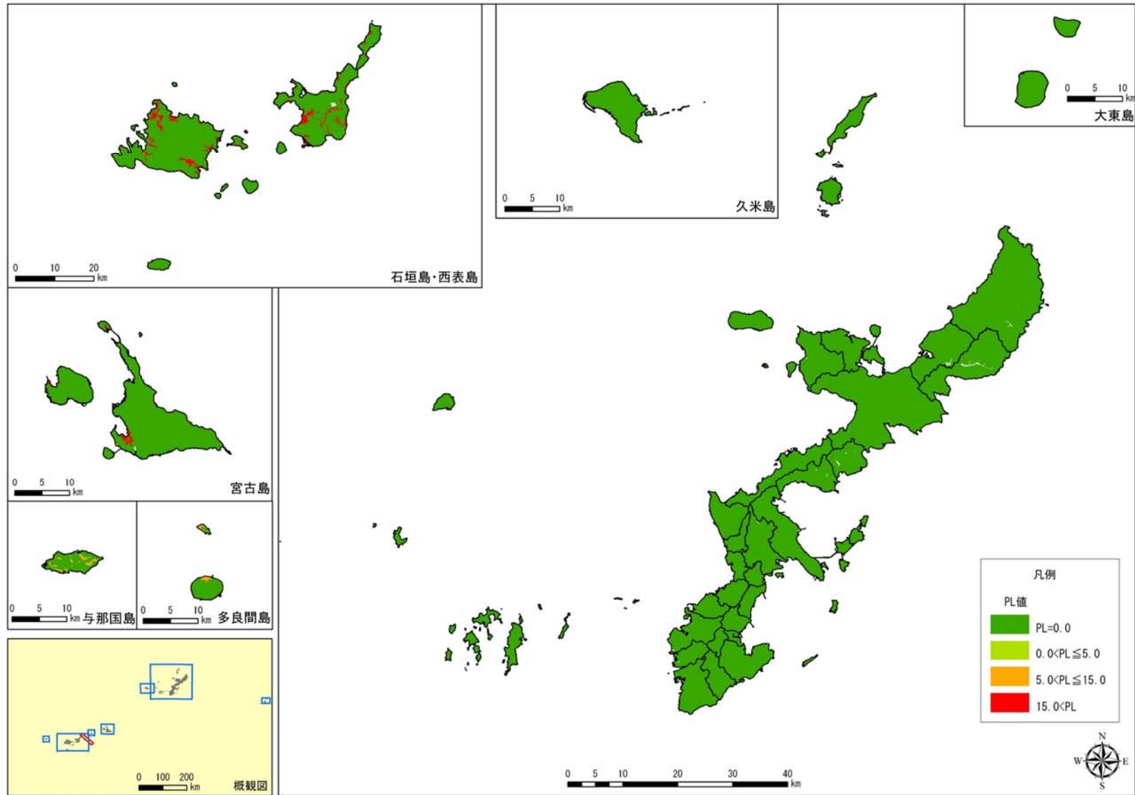
図 2.2-2(13) 石垣島東方沖地震の液状化危険度(PL 値)分布
