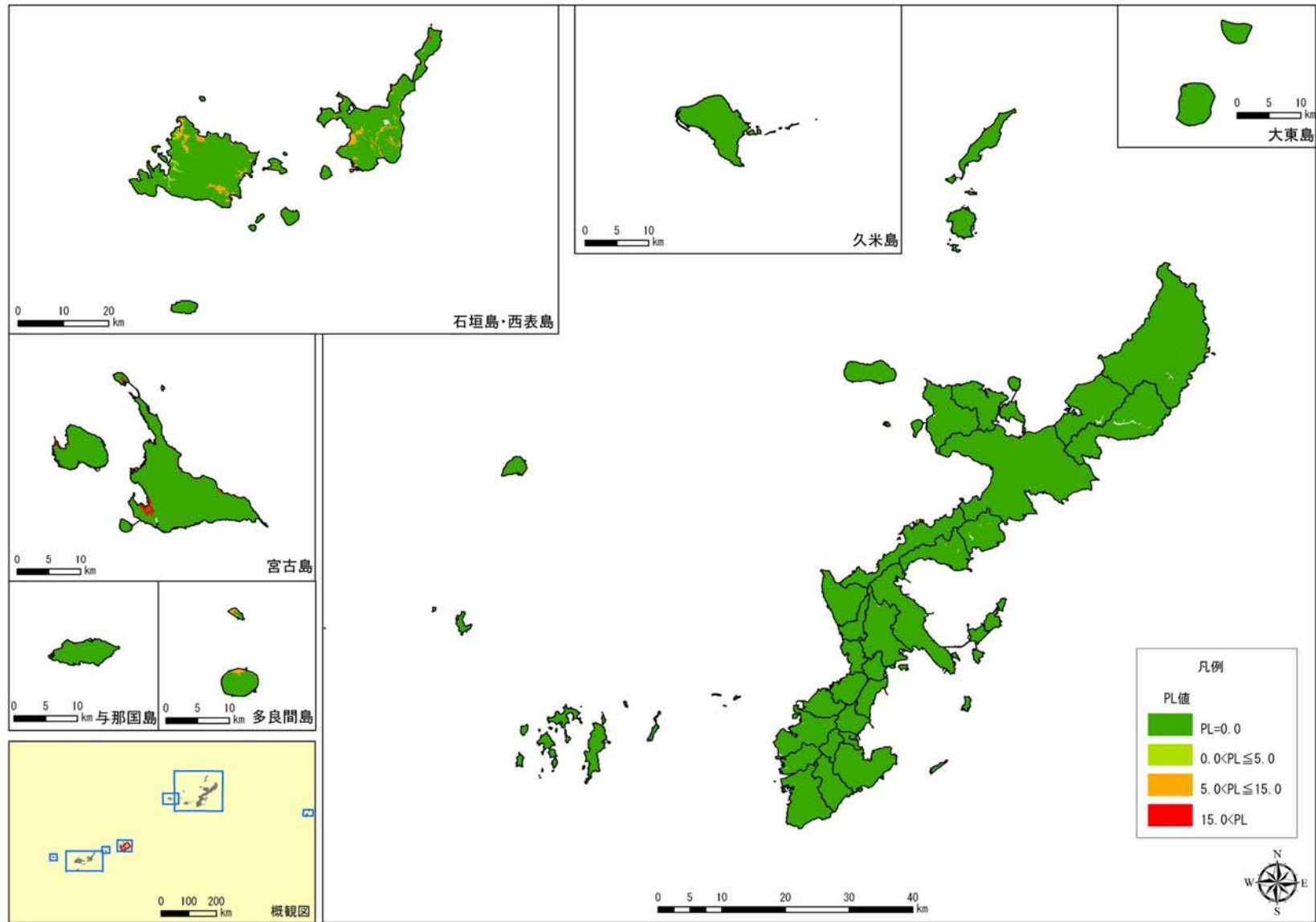
図 2.2-2(23) 宮古島スラブ内地震の液状化危険度(PL 値)分布
