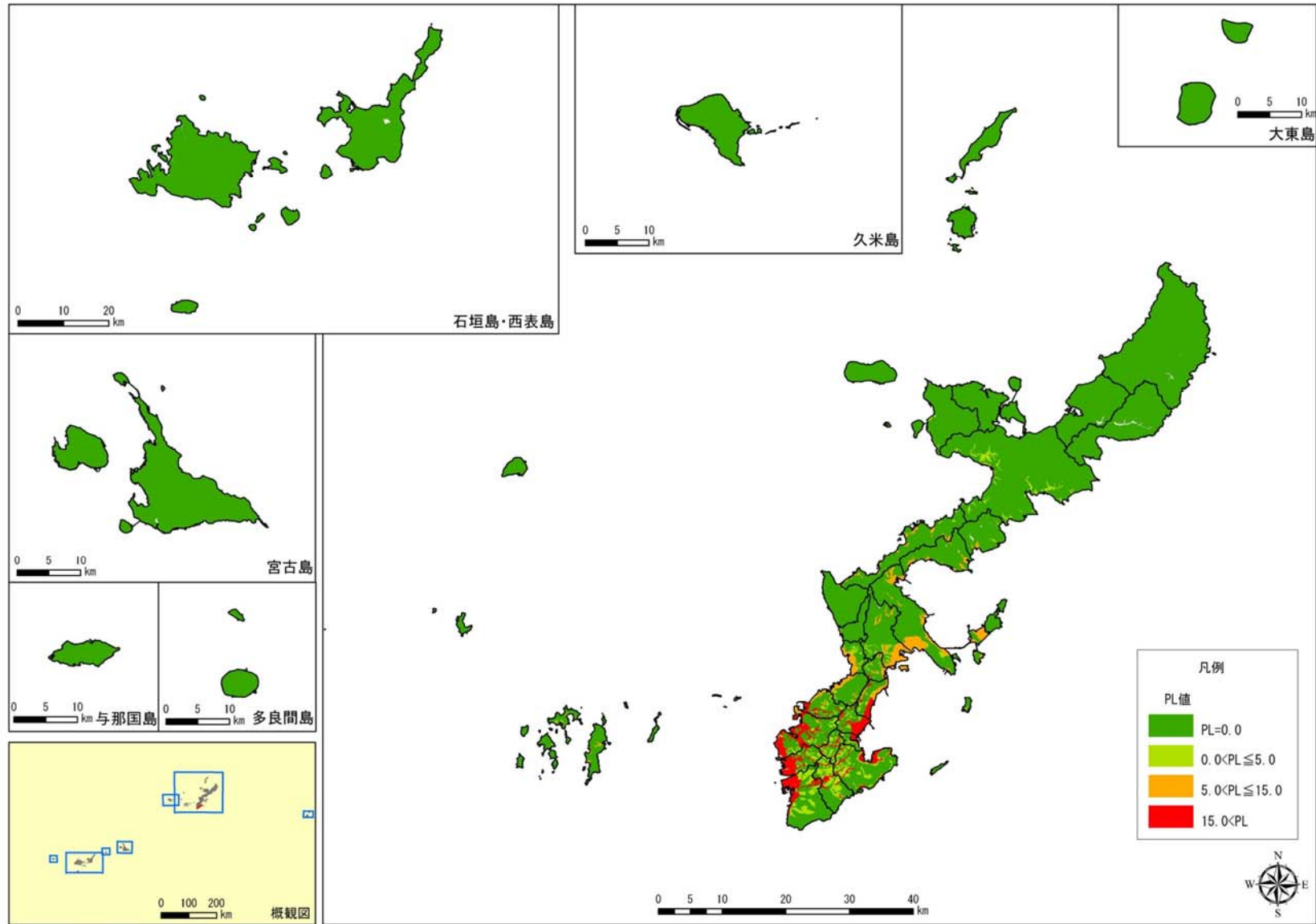
図 2.2-2(1) 沖縄本島南部断層系による地震の液状化危険度(PL 値)分布
