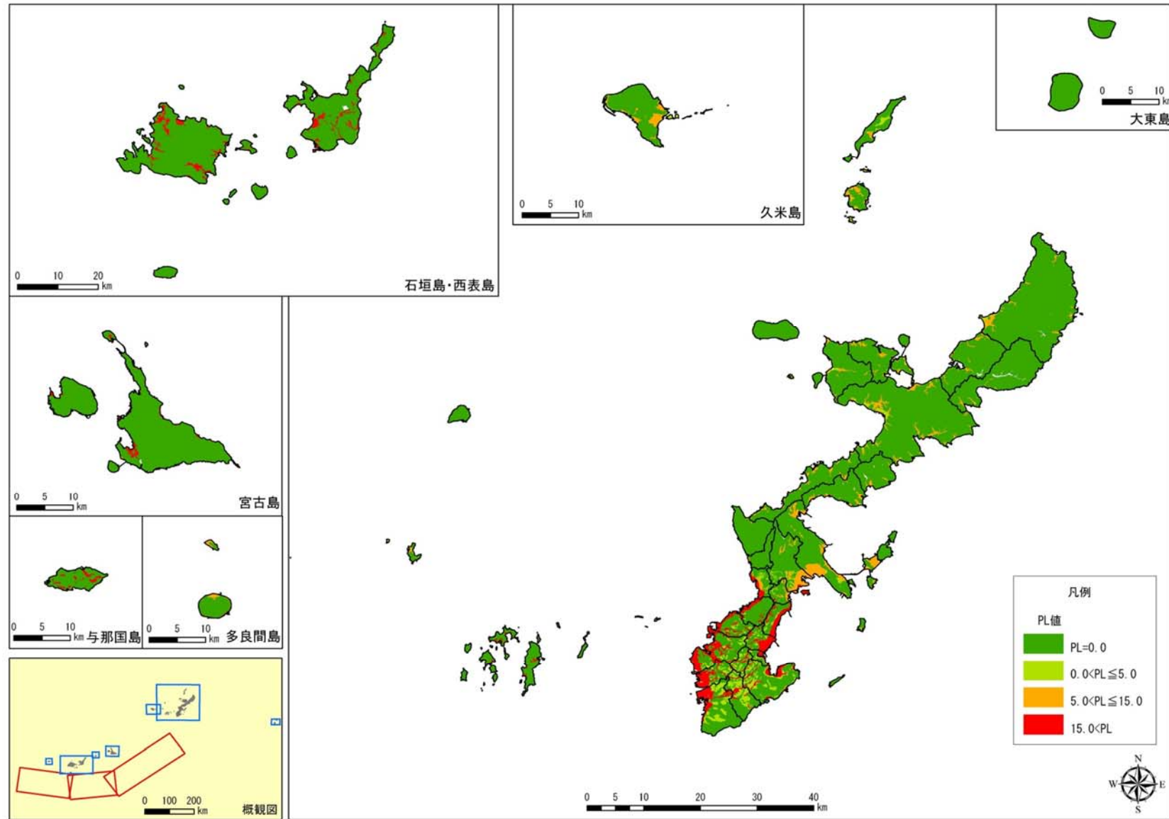
図 2.2-2(21) 八重山諸島南方沖地震3連動の液状化危険度(PL値)分布
