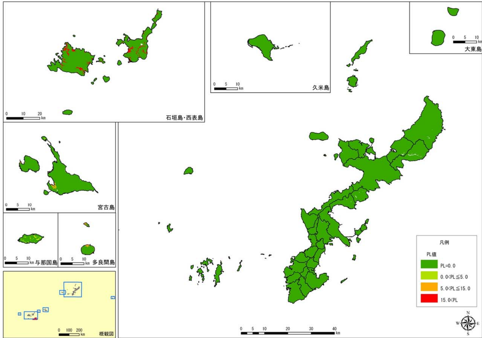
図 2.2-2(12) 石垣島南方沖地震の液状化危険度(PL 値)分布
