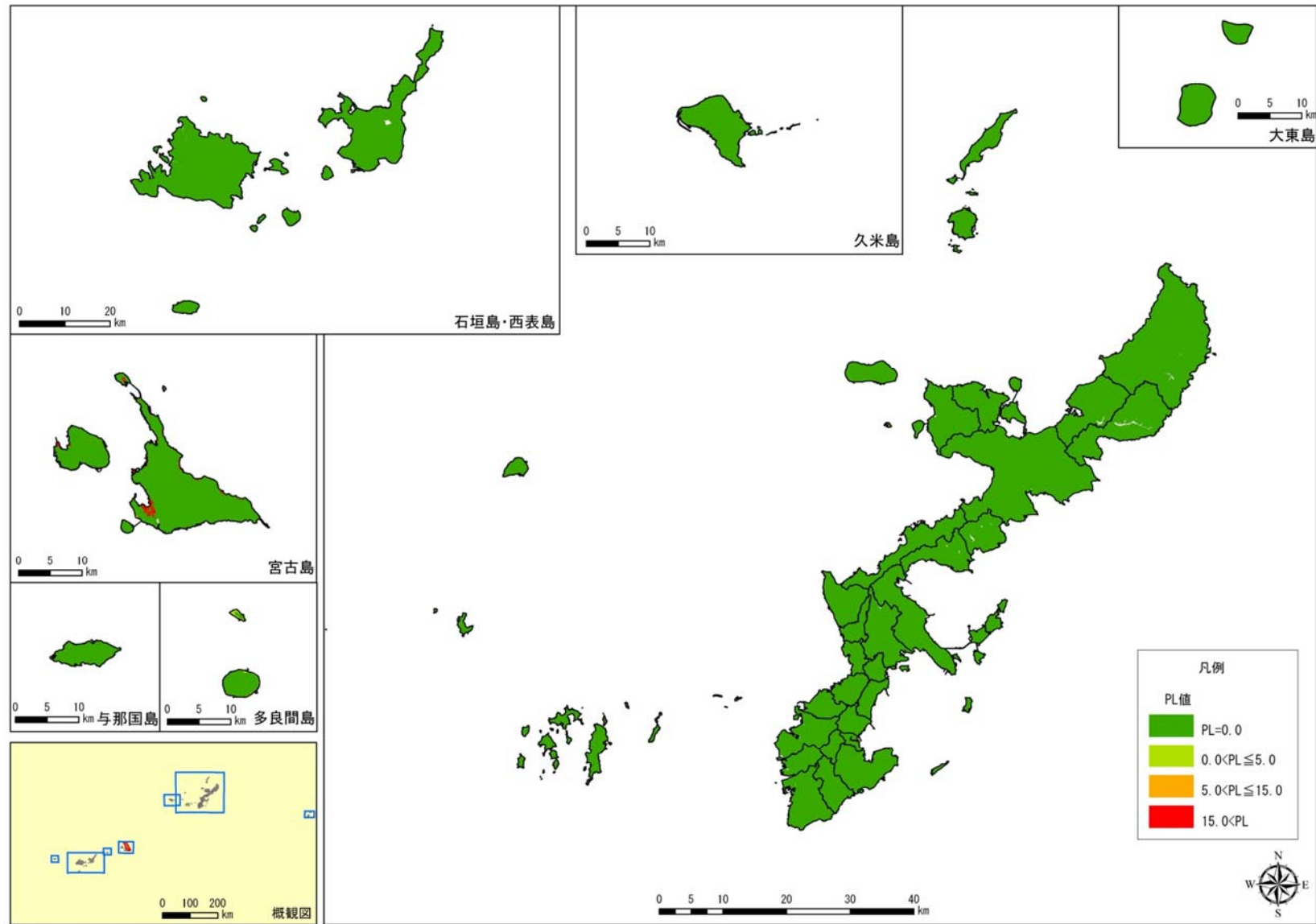
図 2.2-2(5) 宮古島断層による地震の液状化危険度(PL 値)分布
