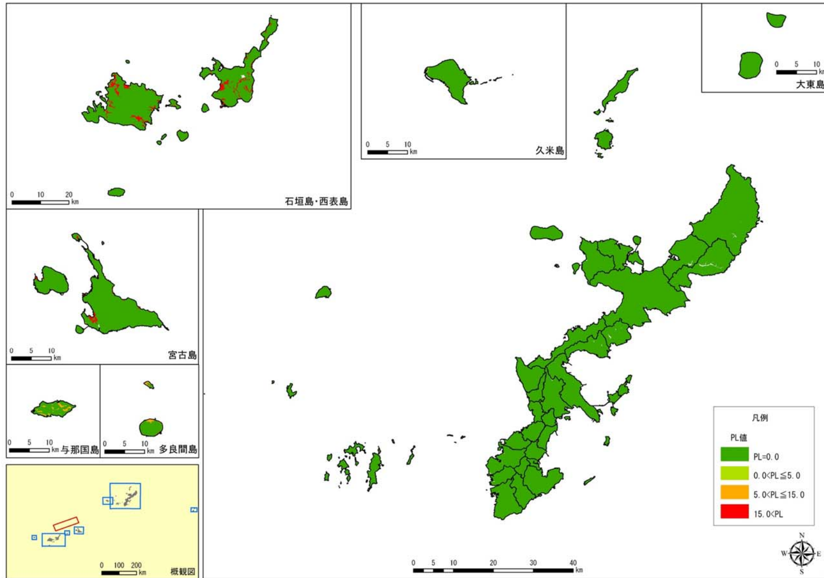
図 2.2-2(16) 多良間島北方沖地震の液状化危険度(PL 値)分布
