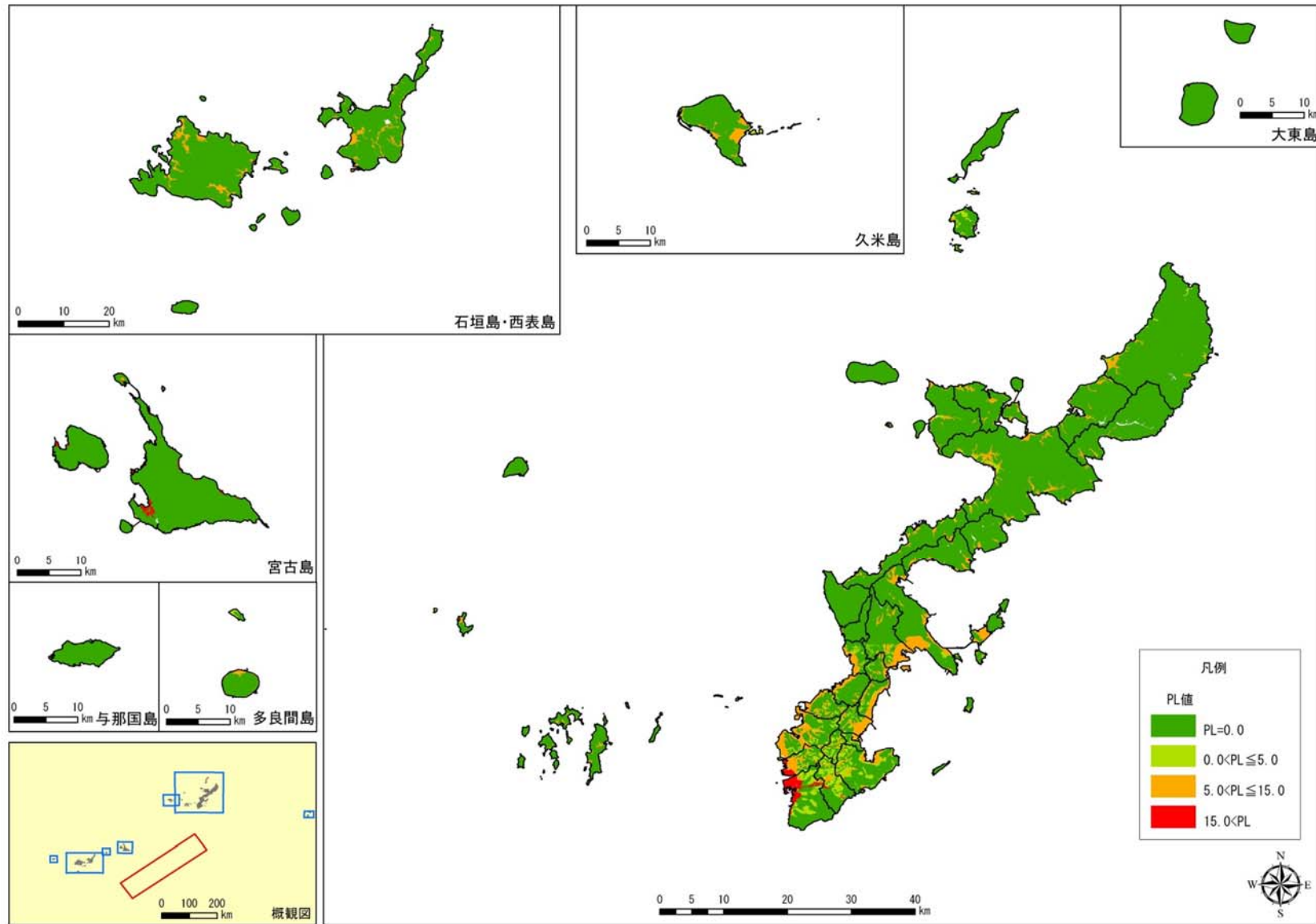
図 2.2-2(9) 八重山諸島南東沖地震の液状化危険度(PL 値)分布
