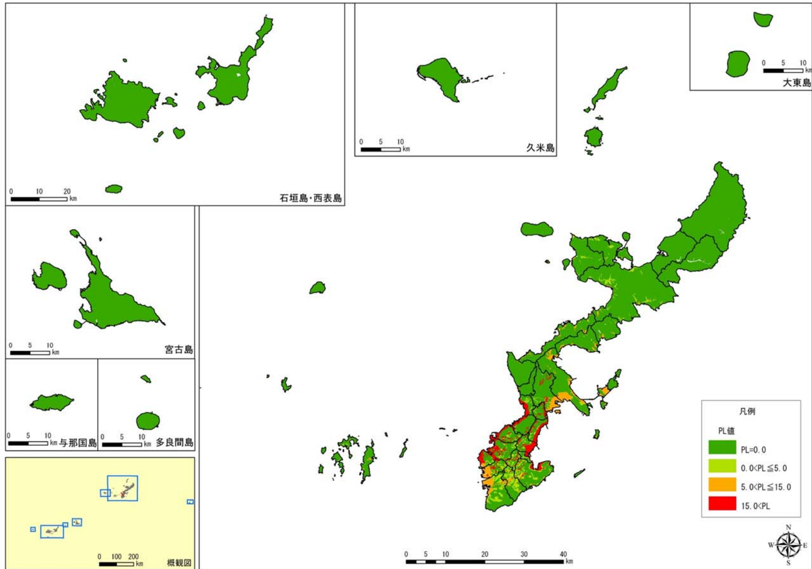
図 2.2-2(2) 伊祖断層による地震の液状化危険度(PL 値)分布
