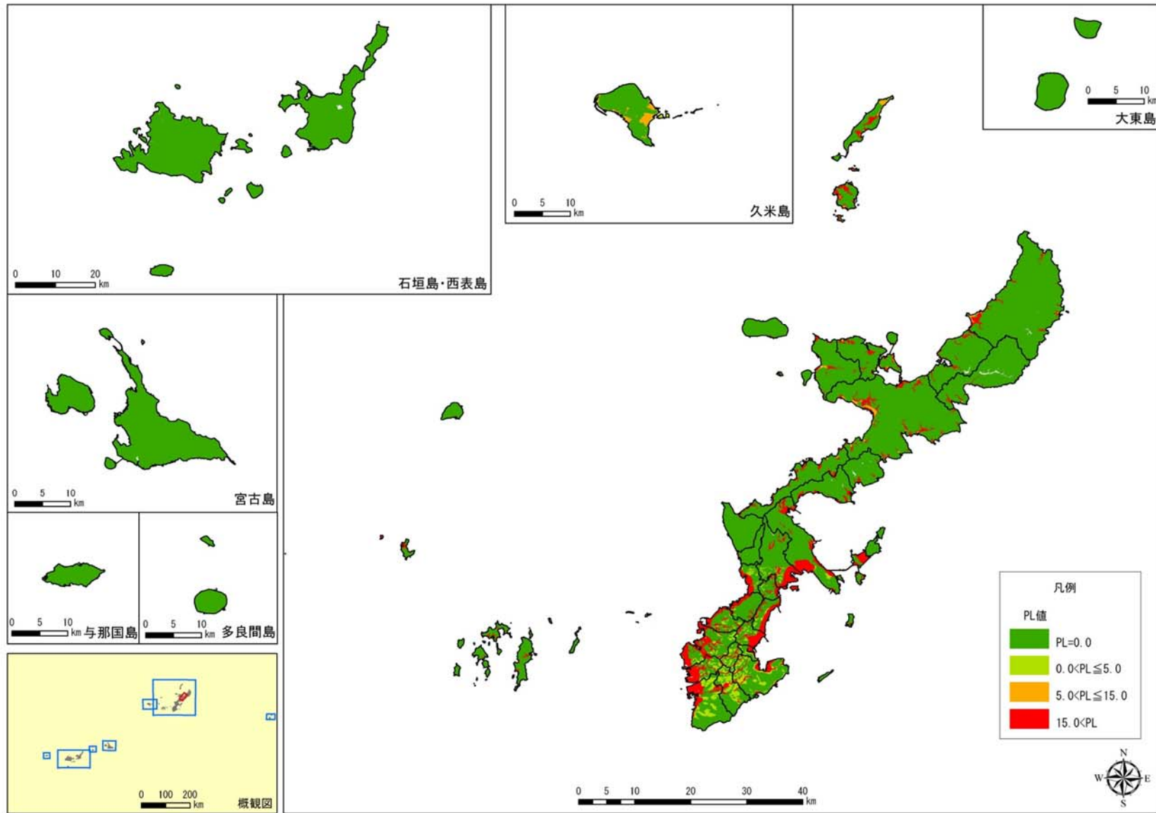
図 2.2-2(22) 沖縄本島北部スラブ内地震の液状化危険度(PL 値)分布
