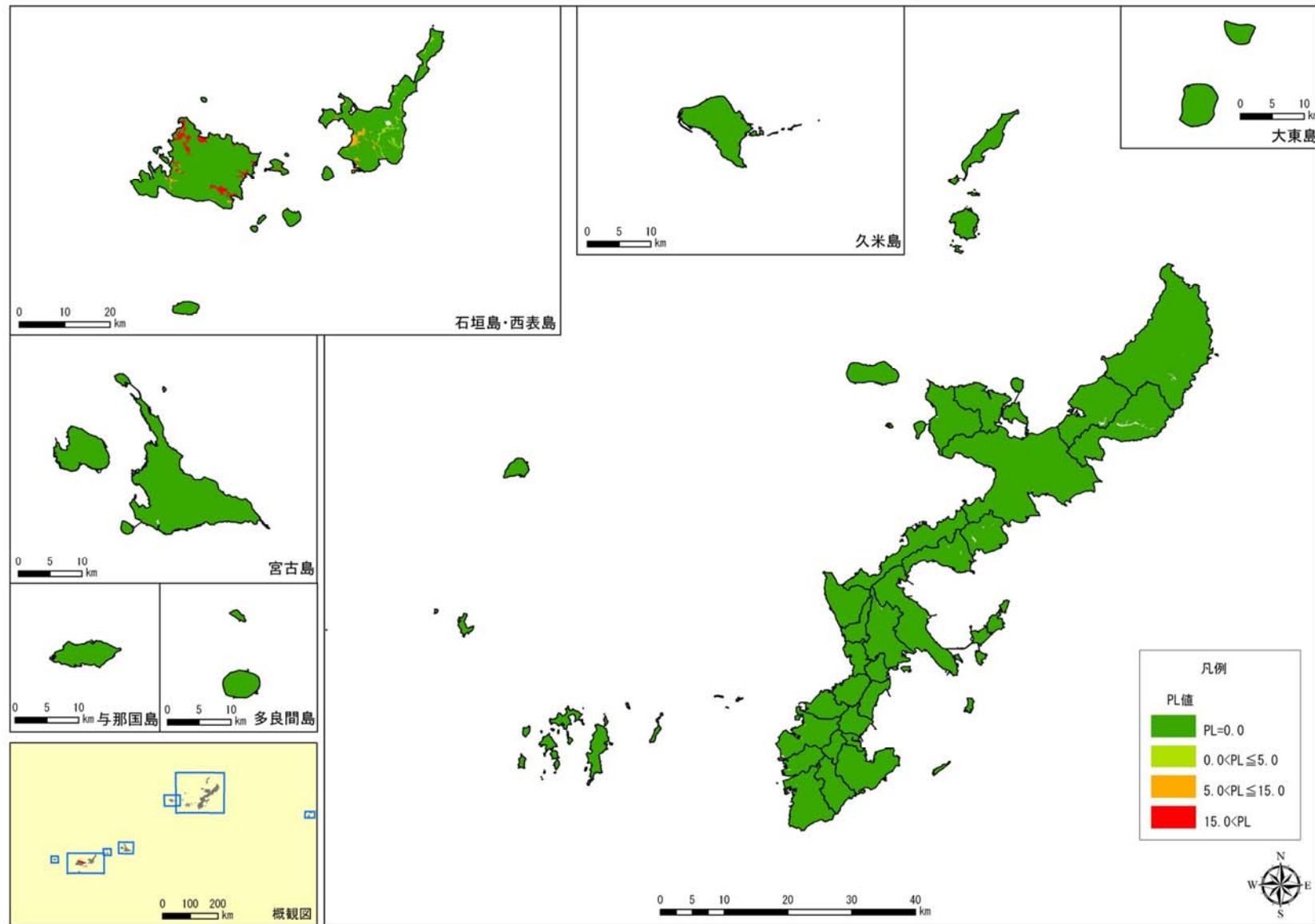
図 2.2-2(6) 西田川ーセナイ湾による地震の液状化危険度(PL 値)分布
