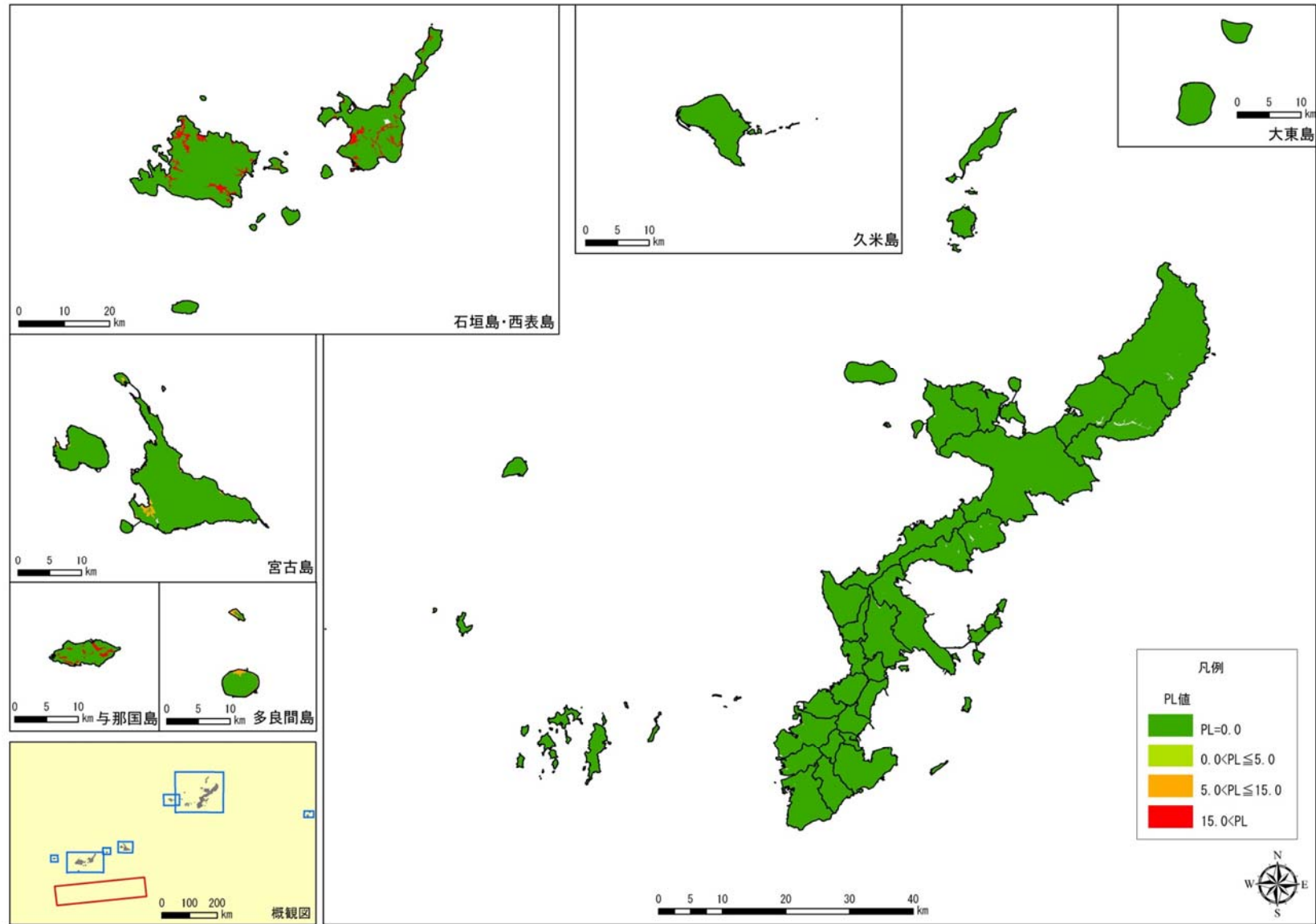
図 2.2-2(8) 八重山諸島南方沖地震の液状化危険度(PL 値)分布
