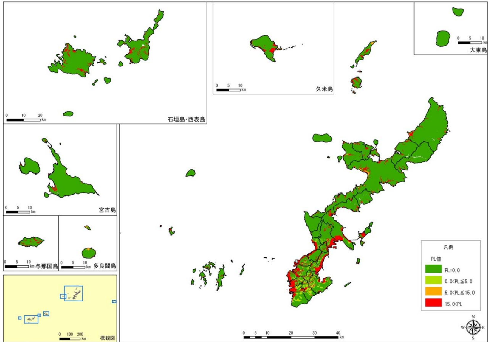
図 2.2-2(25) 一律地震動による地震の液状化危険度(PL 値)分布
