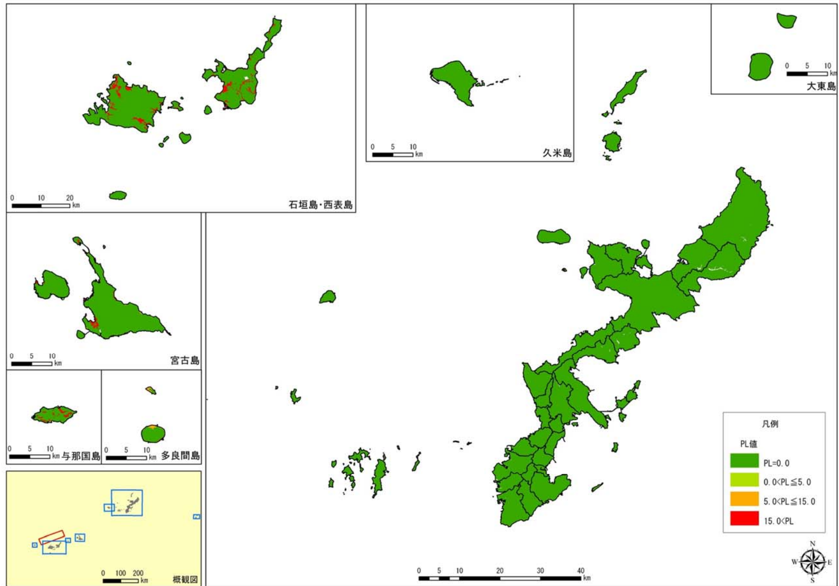
図 2.2-2(15) 石垣島北方沖地震の液状化危険度(PL 値)分布
