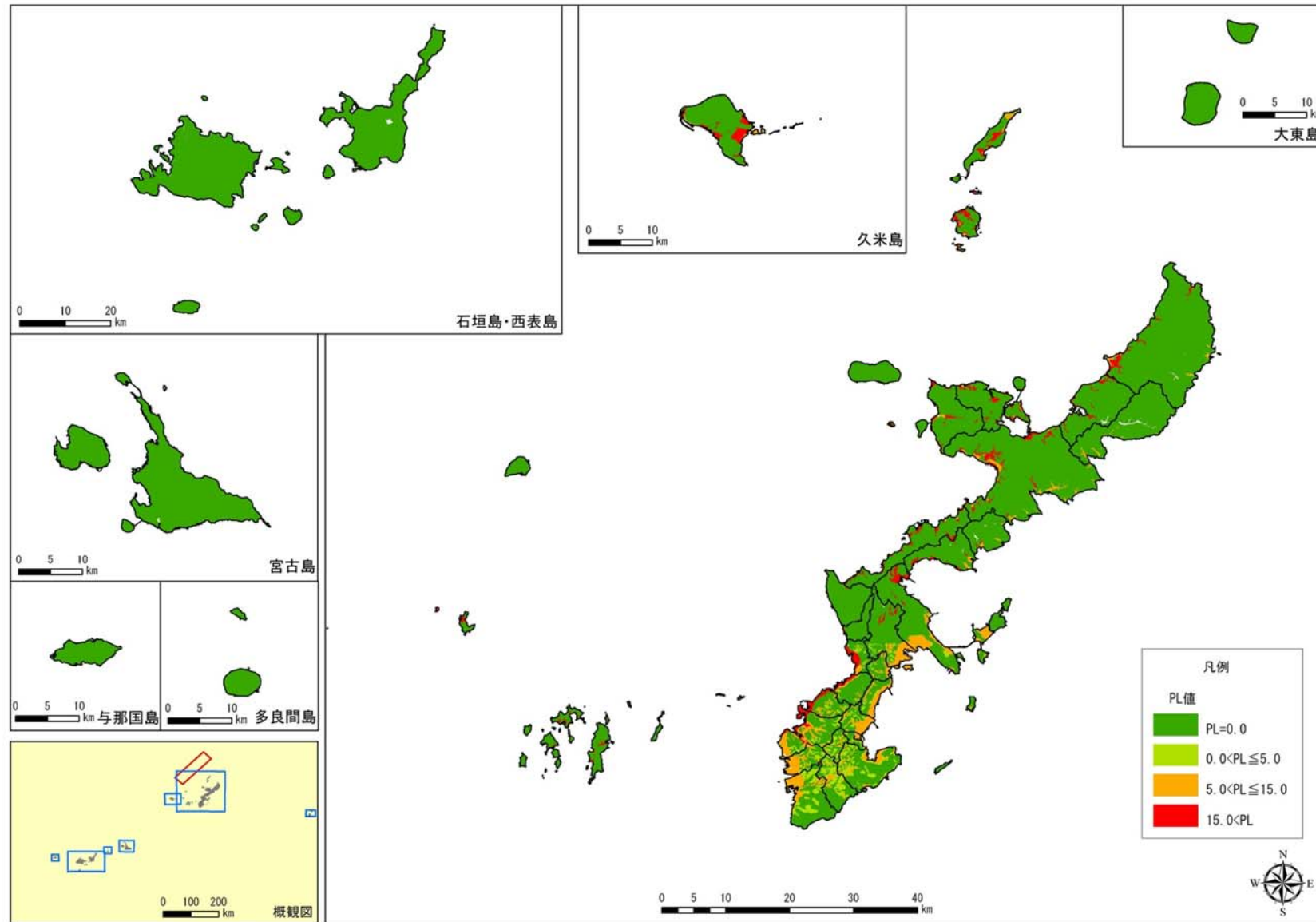
図 2.2-2(19) 沖縄本島北西沖地震の液状化危険度(PL 値)分布
