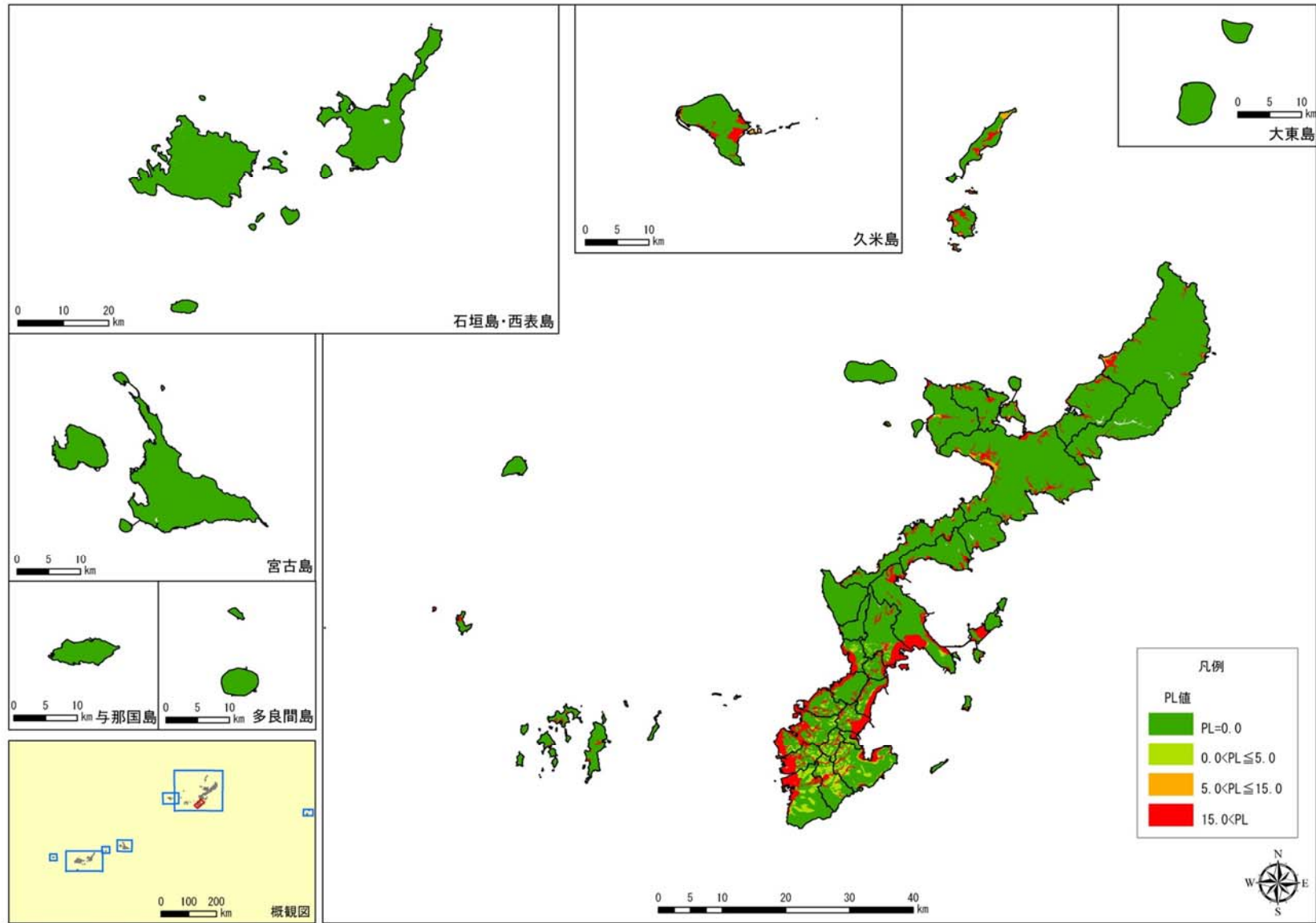
図 2.2-2(4) 沖縄本島南部スラブ内地震の液状化危険度(PL 値)分布
