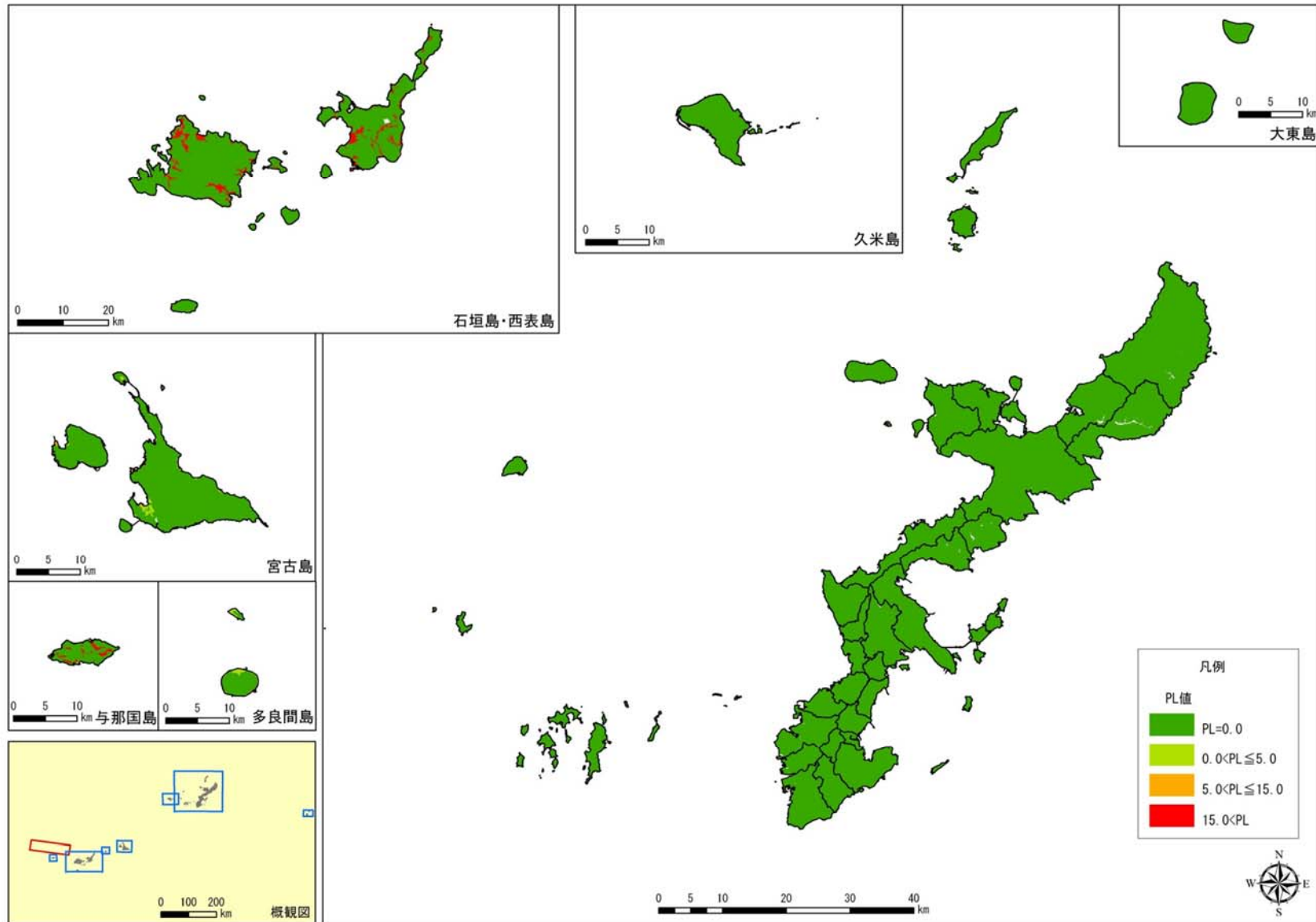
図 2.2-2(14) 与那国島北方沖地震の液状化危険度(PL 値)分布
