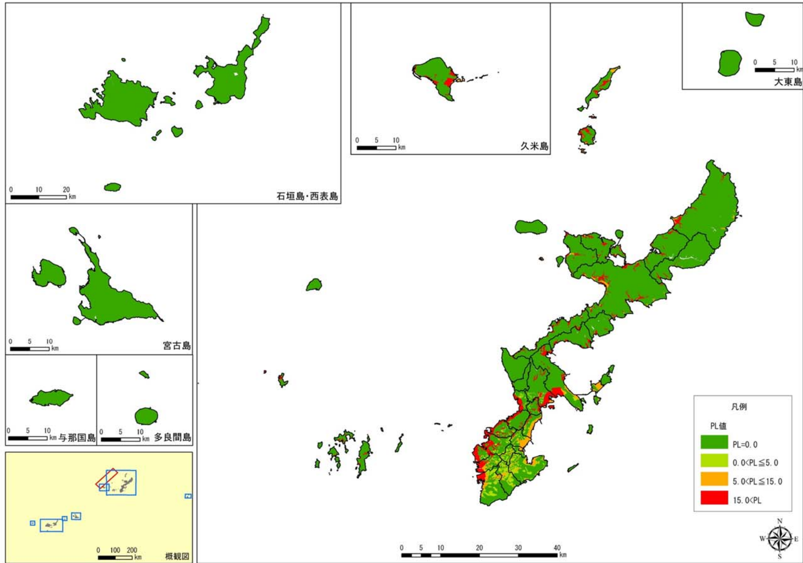
図 2.2-2(18) 久米島北方沖地震の液状化危険度(PL 値)分布
