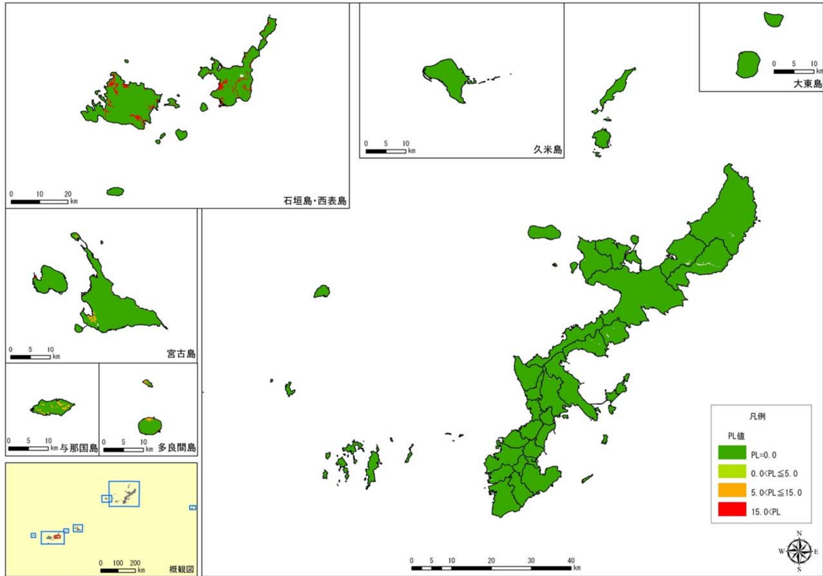
図 2.2-2(24) 石垣島スラブ内地震の液状化危険度(PL 値)分布
