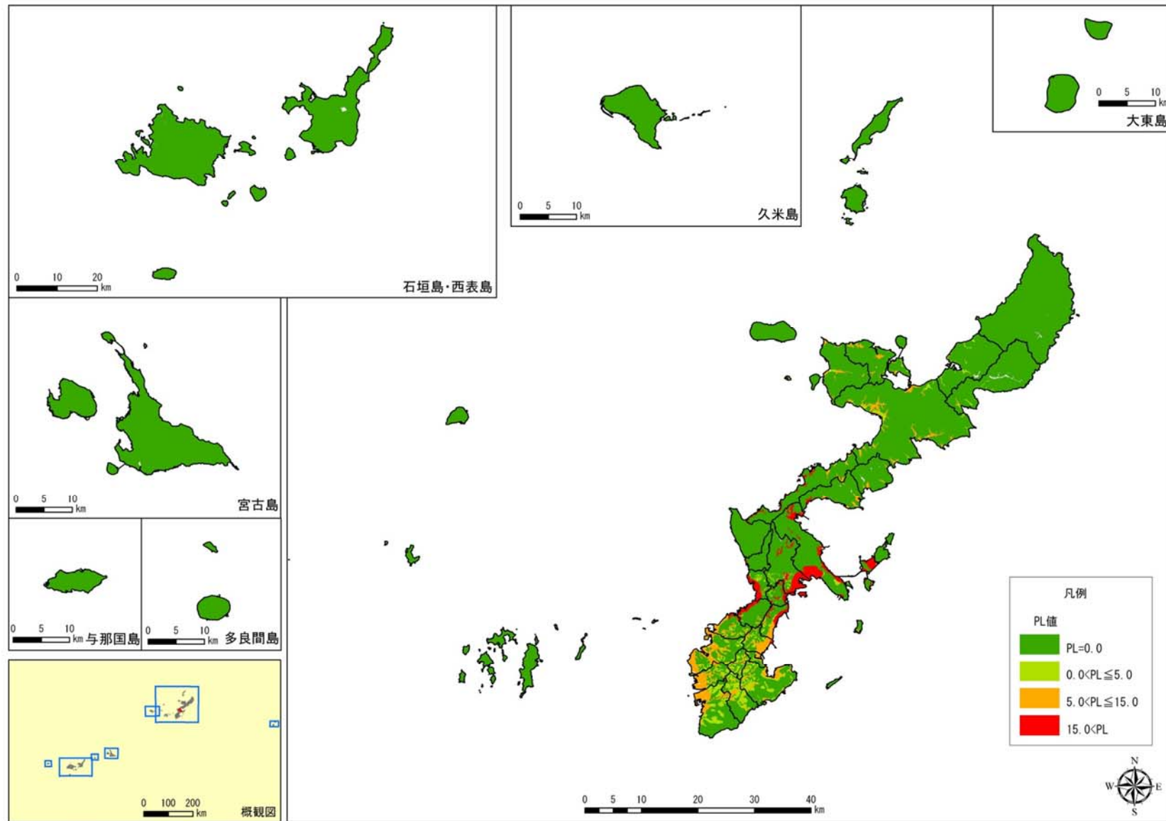
図 2.2-2(3) 石川－具志川断層系による地震の液状化危険度(PL 値)分布
