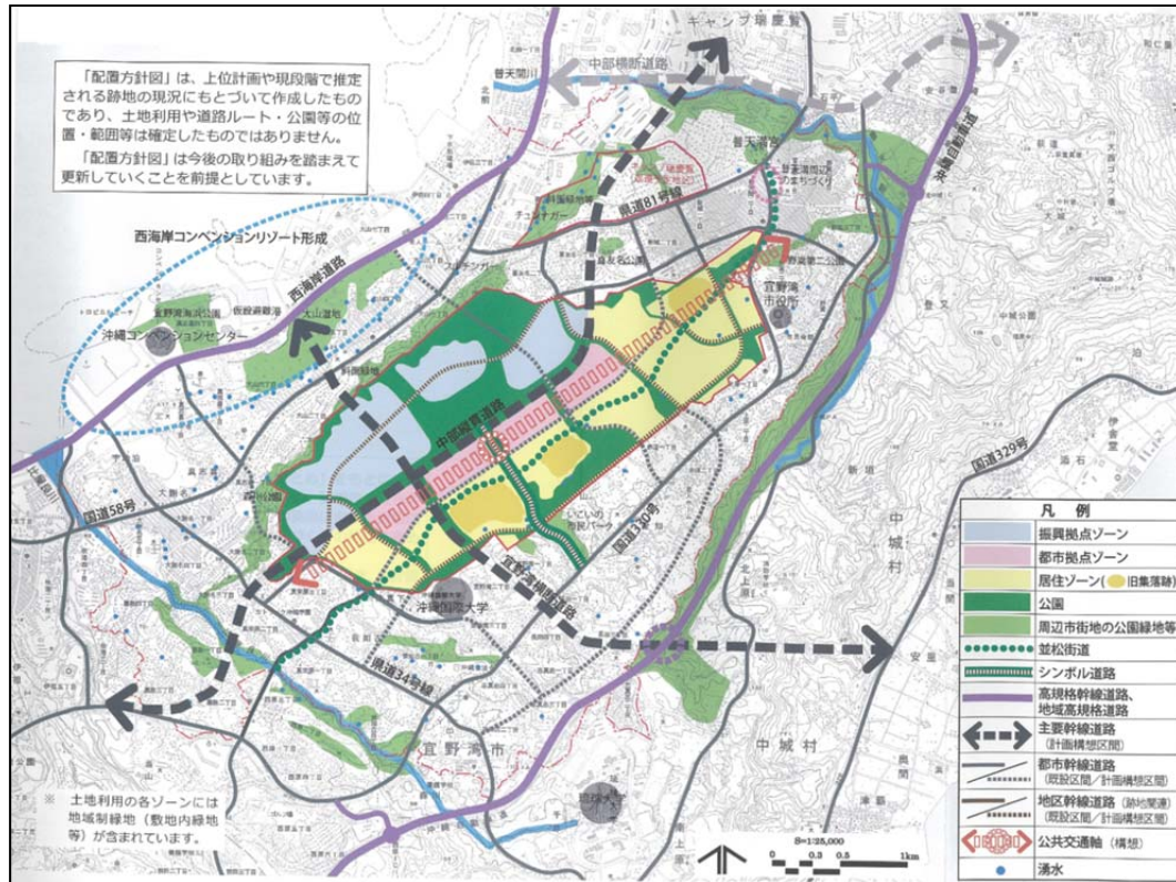
図 2-17 配置方針図
