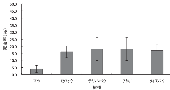
図 - 3 死虫率
