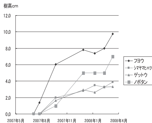
図-2 平均樹高
