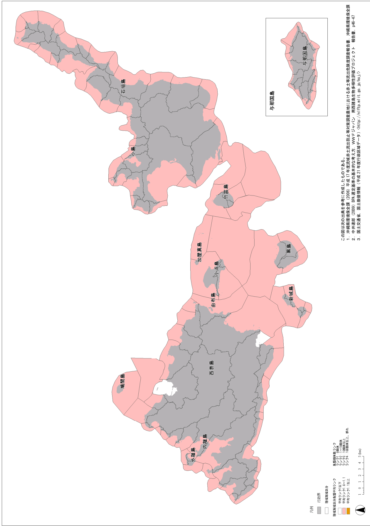
図 4-1-3 2. マンタ法による魚類の陸域海域区分毎の平均ランク (ヒロサ一)
