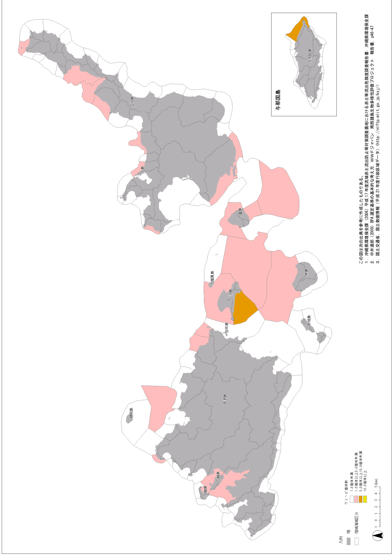
図4-1-35. マンタ法によるウミヘビ類の陸域海域区分毎の合計記録個体数
