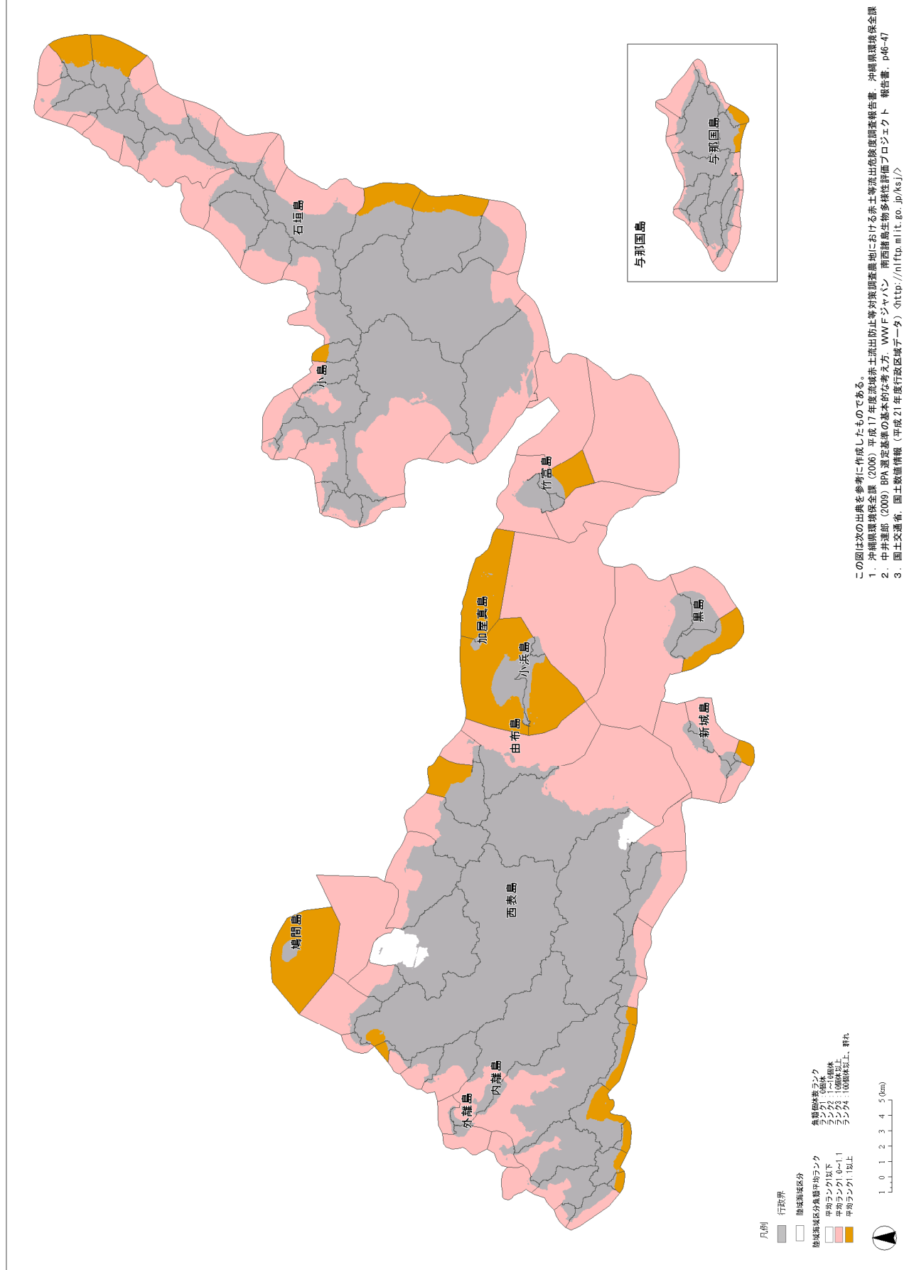
図4-1-28. マンタ法による魚類の陸域海区域毎の平均ランク (カハジャー)
