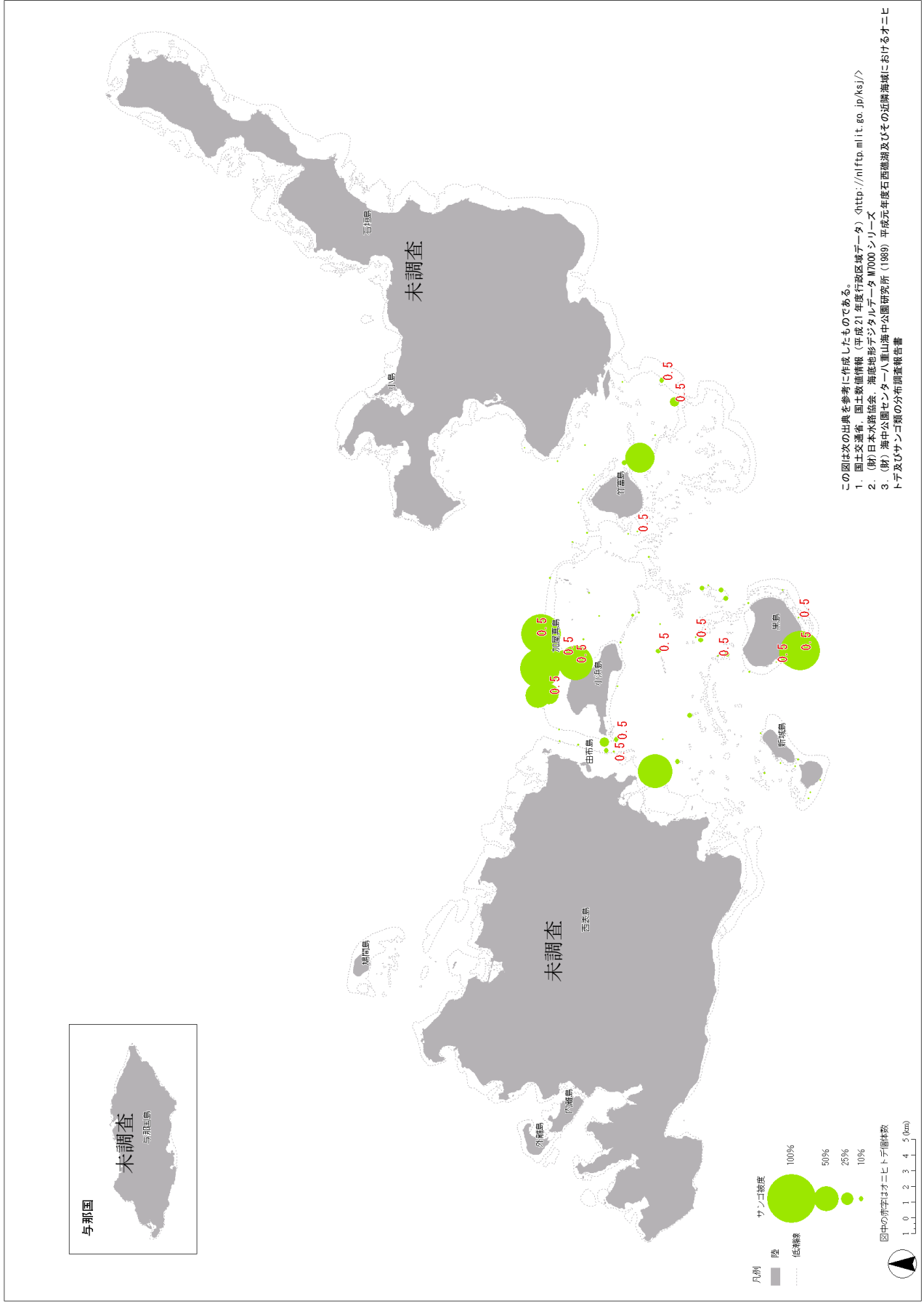
図 4-2-4-6. 1989 年に八重山地域で実施された調査のサンゴ被度とオニヒトデ個体数.
