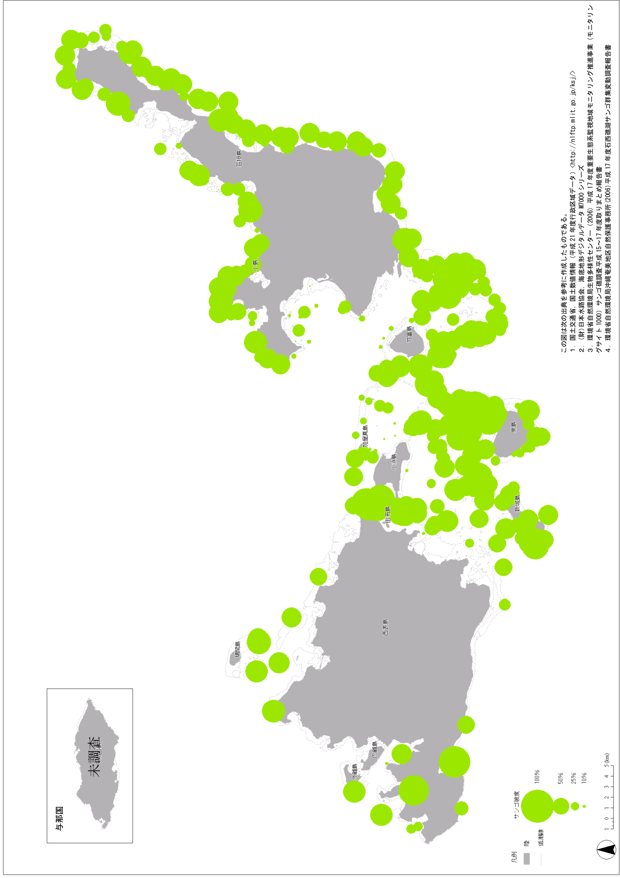
図 4-2-30. 2004 年に八重山地域で実施された簡易遊泳調査のサンゴ被度.
