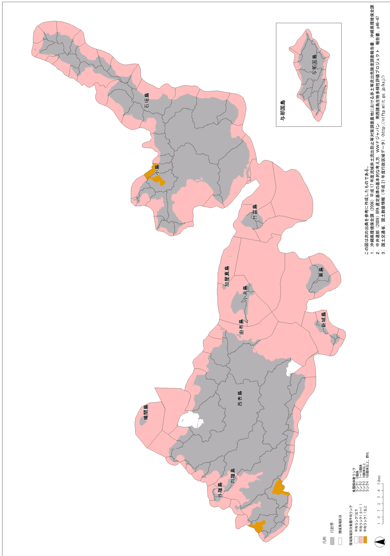
図4-1-2-6. マンタ法による魚類の陸域海域区分毎の平均ランク (タマノシマ)
