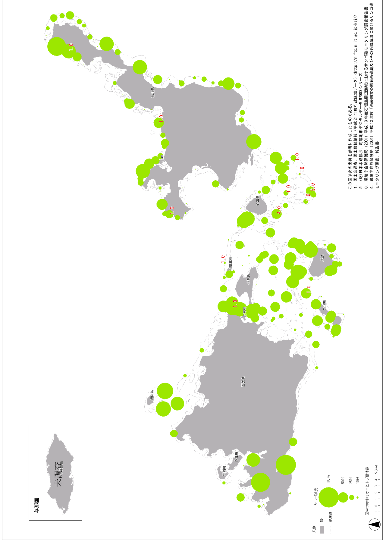
図 4-2-5-8. 2001 年に八重山地域で実施された調査のサンゴ被度とオニヒトデ個体数。
