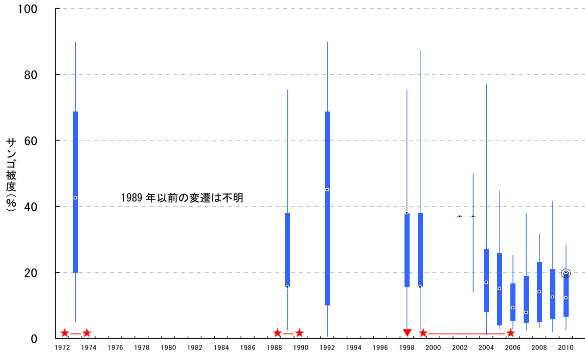
図 2-5-1. 慶良間地域におけるサンゴ被度の変遷と主要なかく乱要因の発生時期. 1989 年以前は、1973 年しか調査が実施されておらず、1974 年から 1988 年間のサンゴ被度の変遷は不明である. 1998 年から 2002 年の変遷は調査が断片的で、サンゴ被度の変遷は断片的である.
