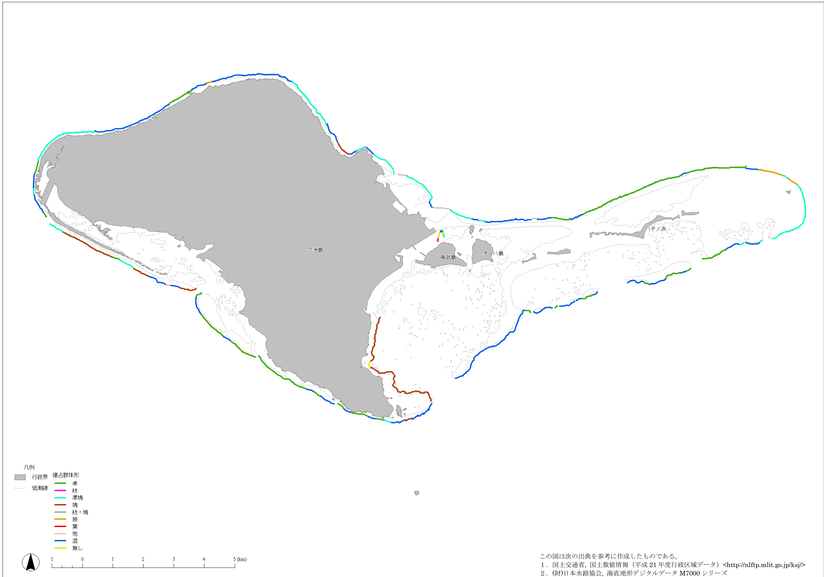
図 3-1-10. マンタ法による調査結果 (優占する群体系)
