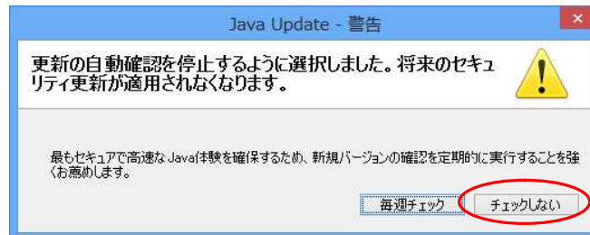
図 3-6 警告画面
