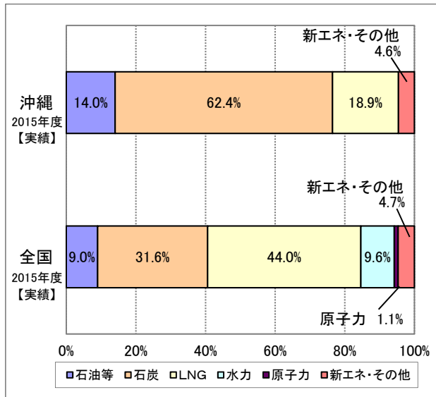
資料: 電気事業連合会「電源別発電電力構成比」及び沖縄電力「沖電統計のあらまし」より作成
