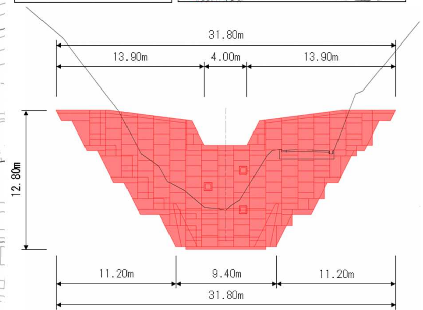
1号砂防堰堤
