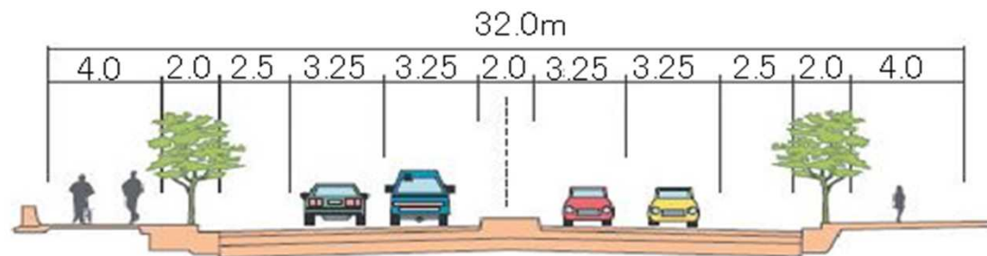
標準断面図
