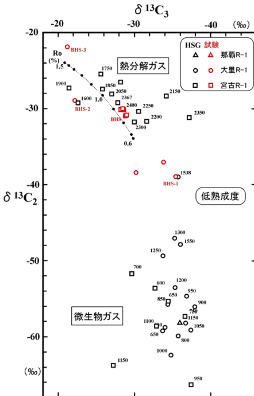
図 2. 2. 31 \delta^{13}C_2 - \delta^{13}C_3 プロット
