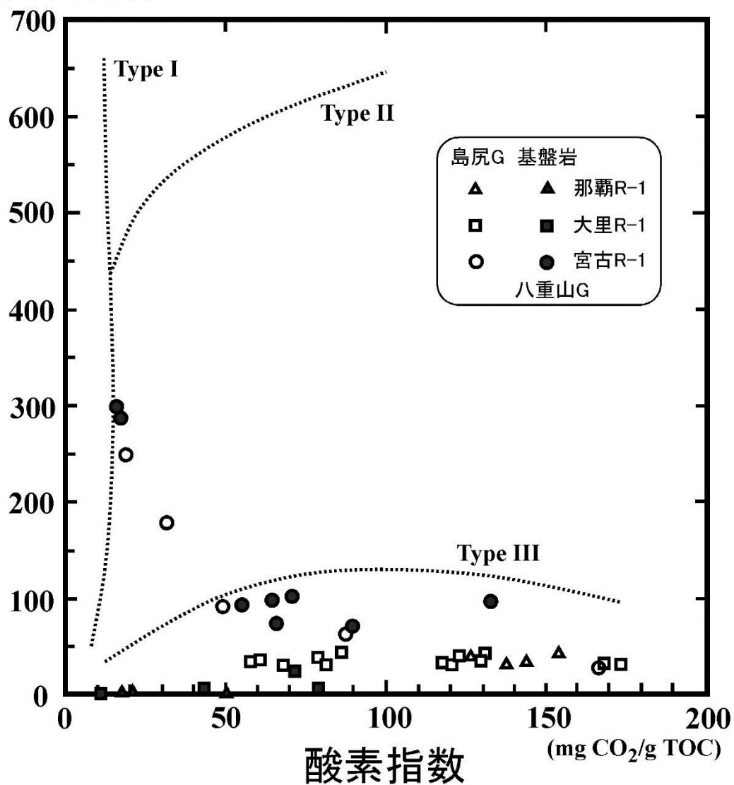
図 2. 2. 26 水素指数－酸素指数プロット
