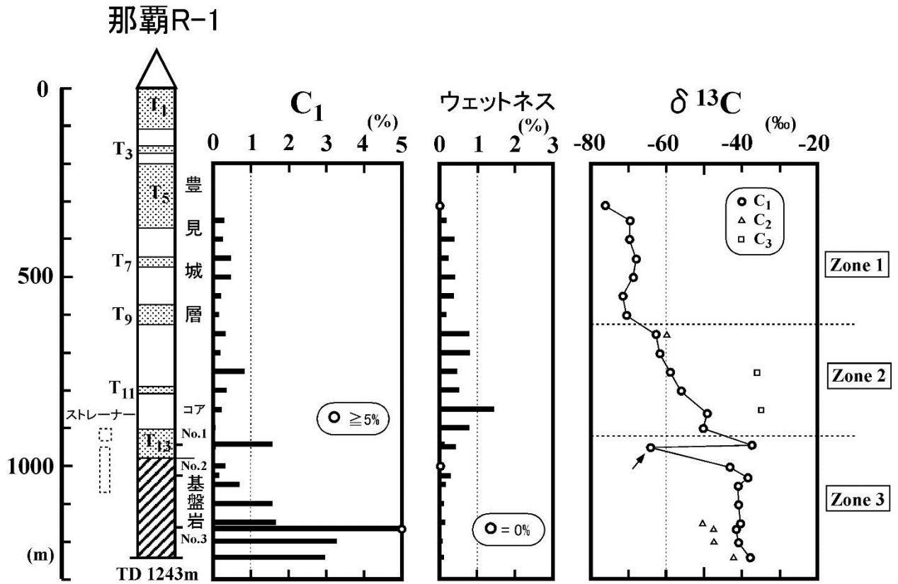
図 2.2.27 ヘッドスペースガスの深度変化 (那覇 R-1)
