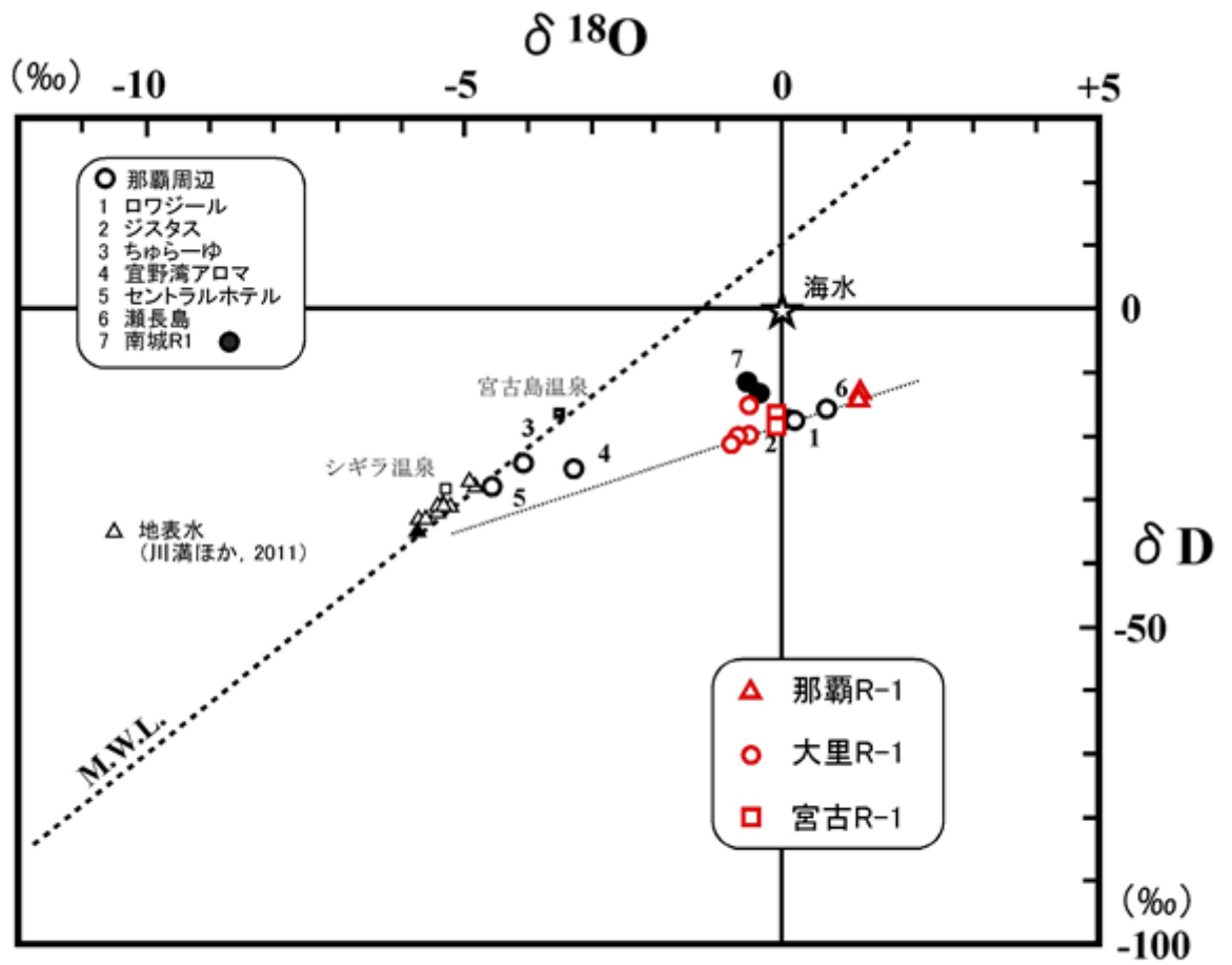
図 2.2.34 地層水の Cl--I-プロット
