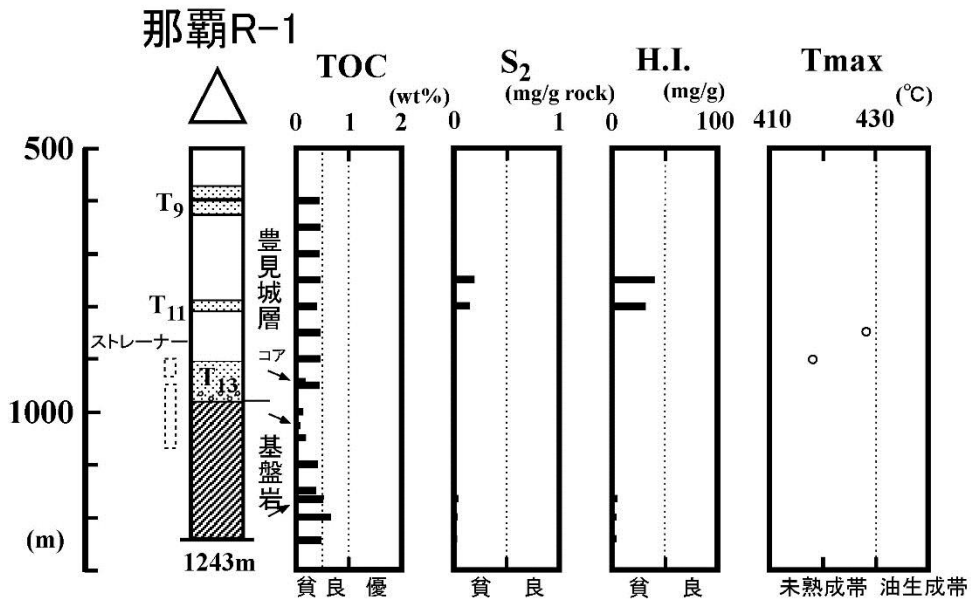
図 2. 2. 23 根源岩評価パラメータの深度変化(那覇 R-1)
