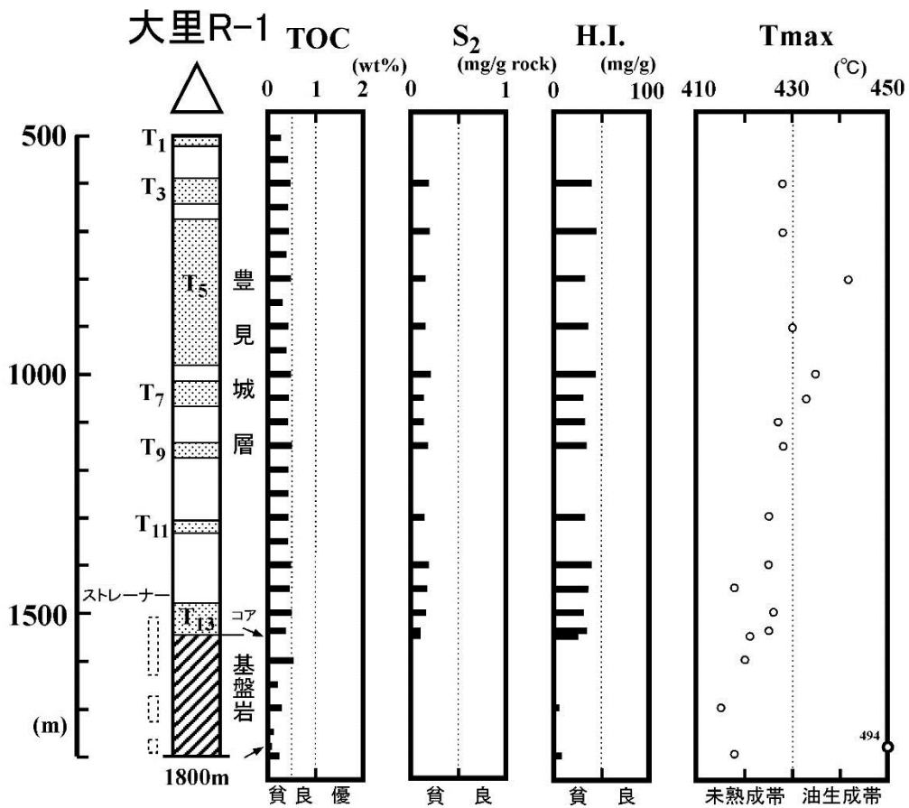
図 2. 2. 24 根源岩評価パラメータの深度変化(大里 R-1)
