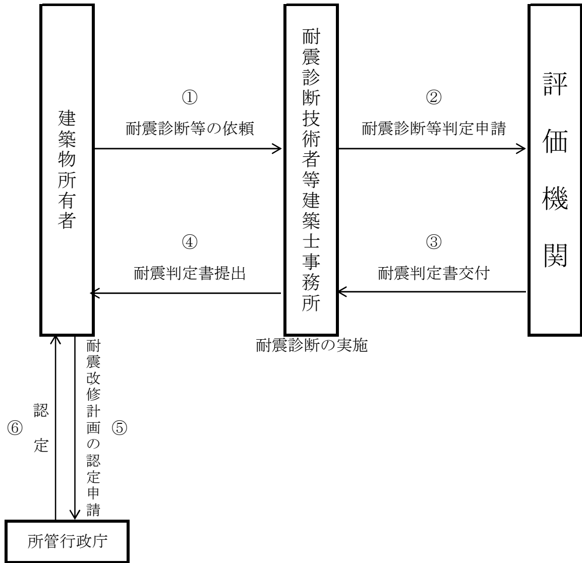
耐震改修計画の認定申請フロー図
