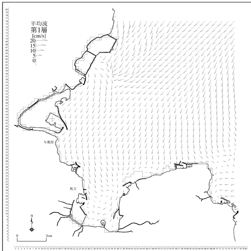
図 3-5-25(7) 将来潮流計算結果 (計画変更あり : 冬季、恒流 (平均流) [第 1 層])
