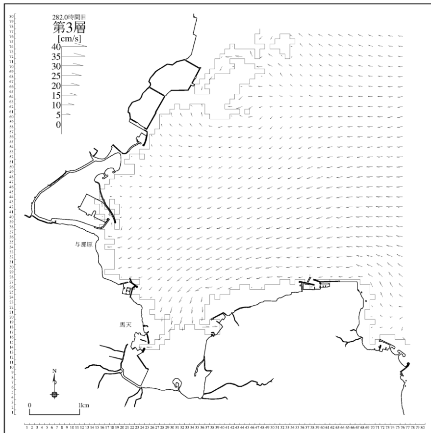
図 3-5-24(3) 将来潮流計算結果（計画変更あり：夏季、上げ潮時[第3層]）
