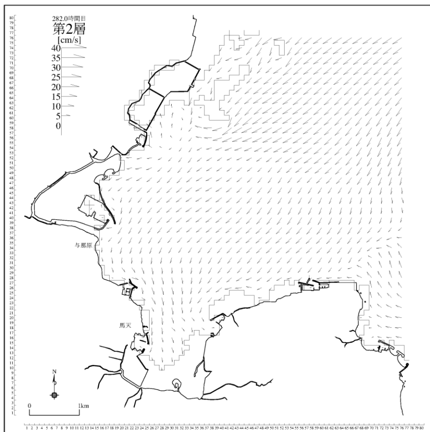
図 3-5-25 (2) 将来潮流計算結果 (計画変更あり：冬季、上げ潮時[第 2 層])
