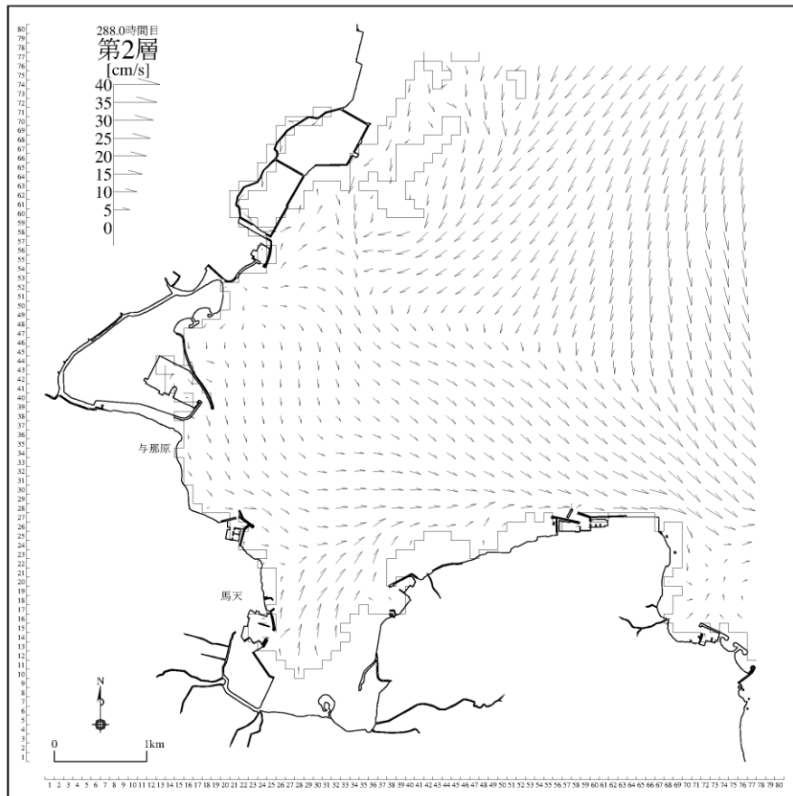
図 3-5-25(5) 将来潮流計算結果（計画変更あり：冬季、下げ潮時[第2層]）
