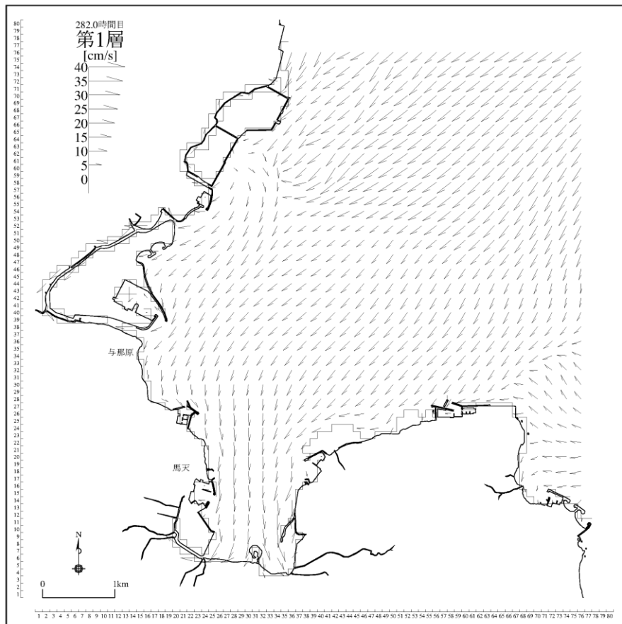
図 3-5-25(1) 将来潮流計算結果（計画変更あり：冬季、上げ潮時[第1層]）
