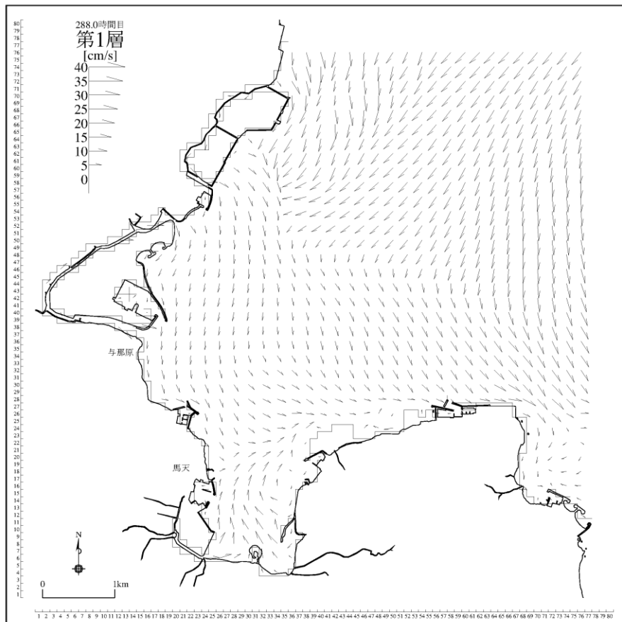
図 3-5-25(4) 将来潮流計算結果（計画変更あり：冬季、下げ潮時[第1層]）
