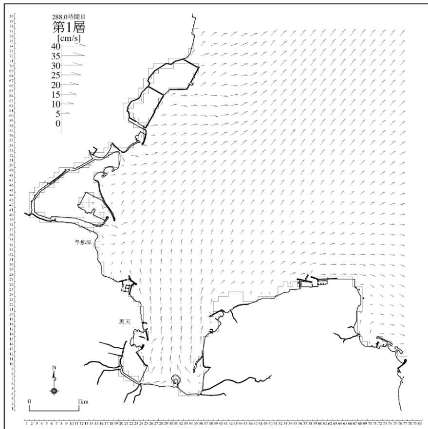
図 3-5-24(4) 将来潮流計算結果（計画変更あり：夏季、下げ潮時[第1層]）
