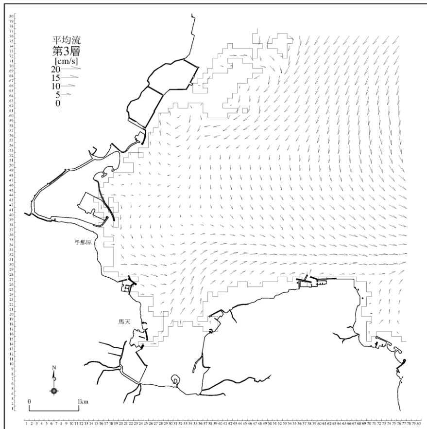
図 3-5-25(9) 将来潮流計算結果 (計画変更あり: 冬季、恒流 (平均流) [第3層])
