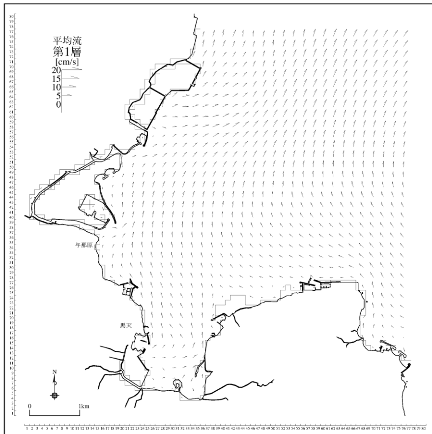
図 3-5-24(7) 将来潮流計算結果 (計画変更あり: 夏季、恒流 (平均流) [第1層])
