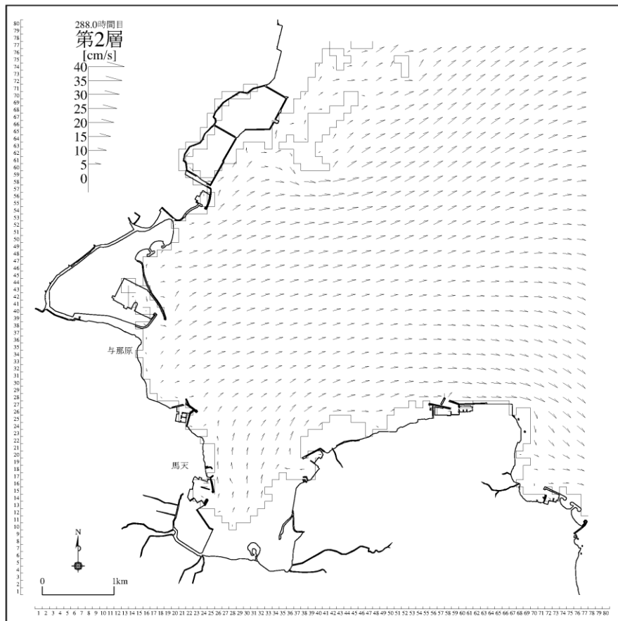
図 3-5-24(5) 将来潮流計算結果（計画変更あり：夏季、下げ潮時[第2層]）
