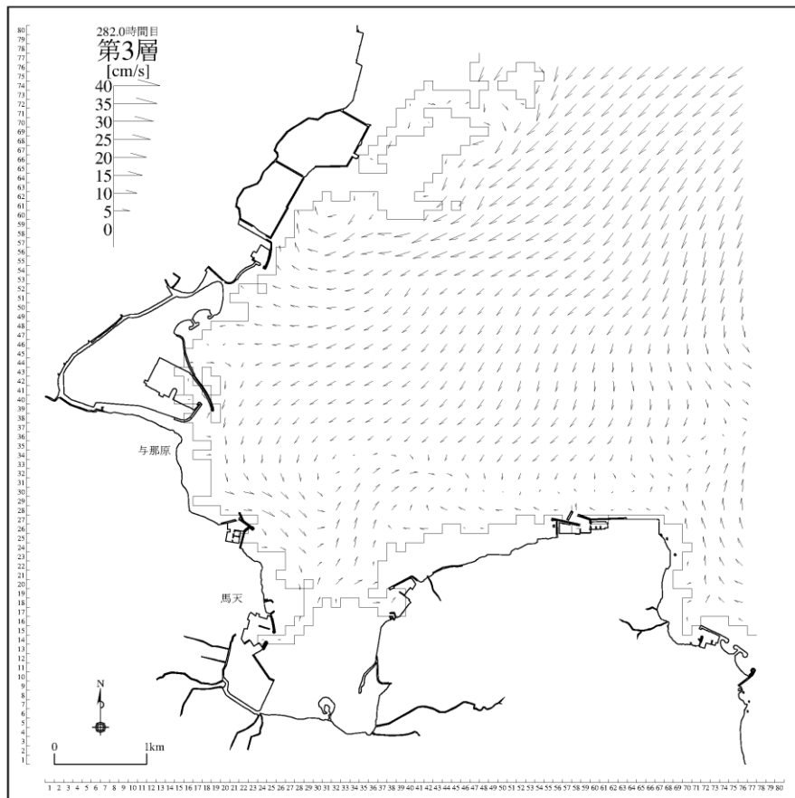
図 3-5-25(3) 将来潮流計算結果（計画変更あり：冬季、上げ潮時[第3層]）
