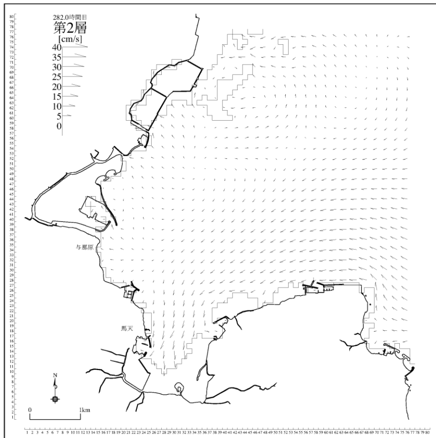
図 3-5-24(2) 将来潮流計算結果 (計画変更あり: 夏季、上げ潮時[第2層])
