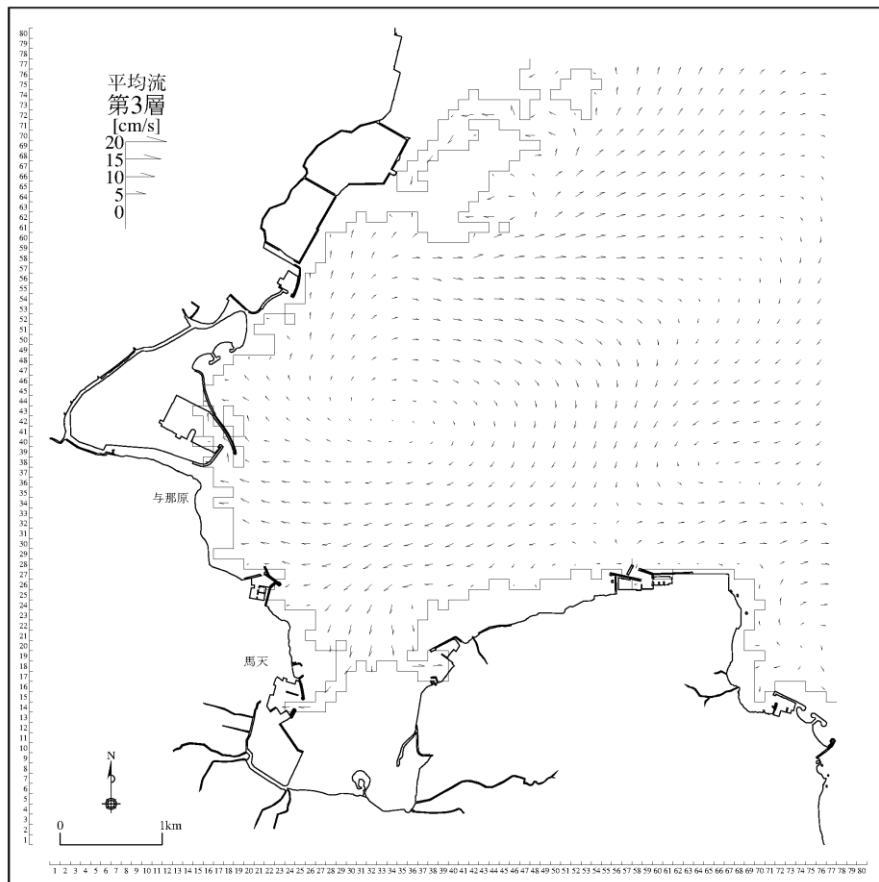
図 3-5-24(9) 将来潮流計算結果 (計画変更あり：夏季、恒流 (平均流) [第3層])
