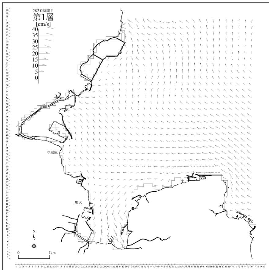
図 3-5-24(1) 将来潮流計算結果（計画変更あり：夏季、上げ潮時[第1層]）
