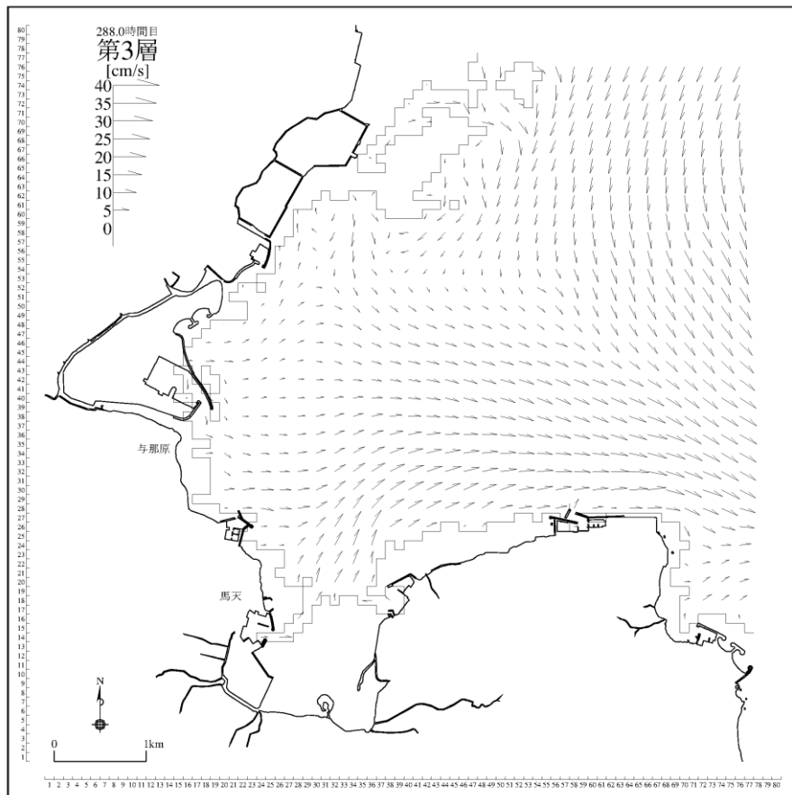
図 3-5-25 (6) 将来潮流計算結果 (計画変更あり: 冬季、下げ潮時[第3層])
