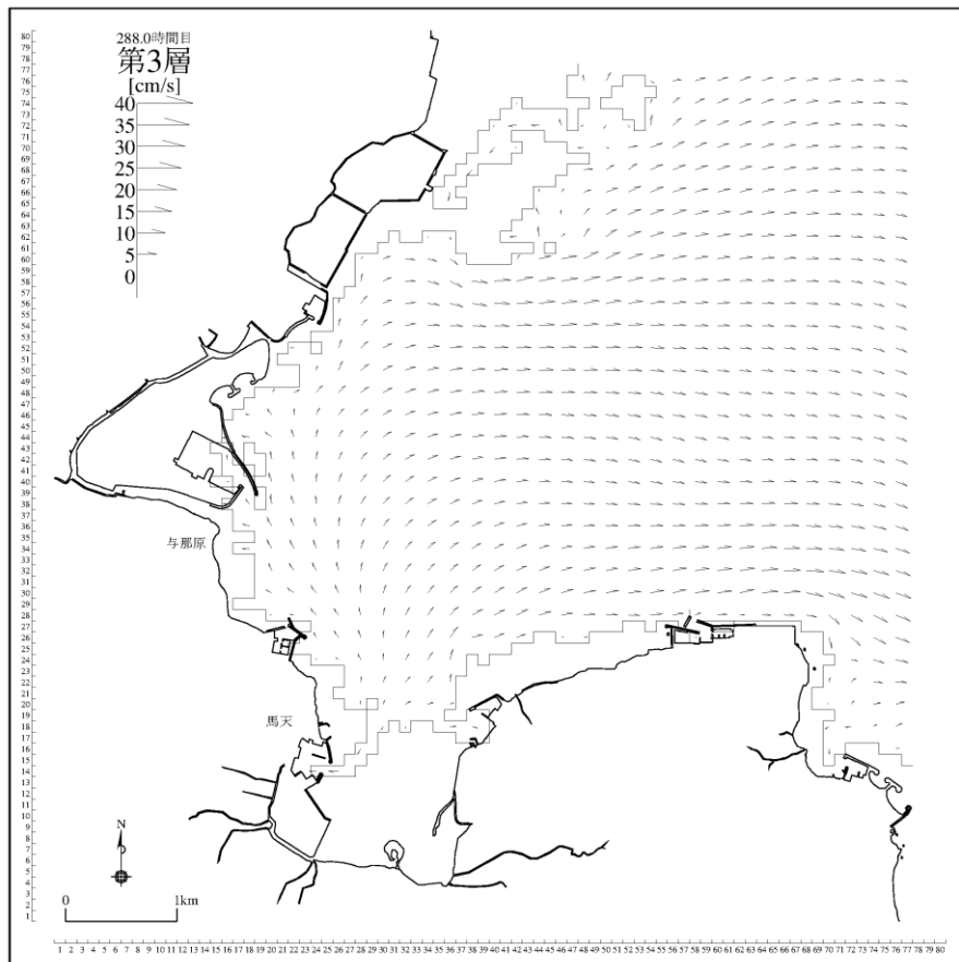
図 3-5-24(6) 将来潮流計算結果（計画変更あり：夏季、下げ潮時[第3層]）
