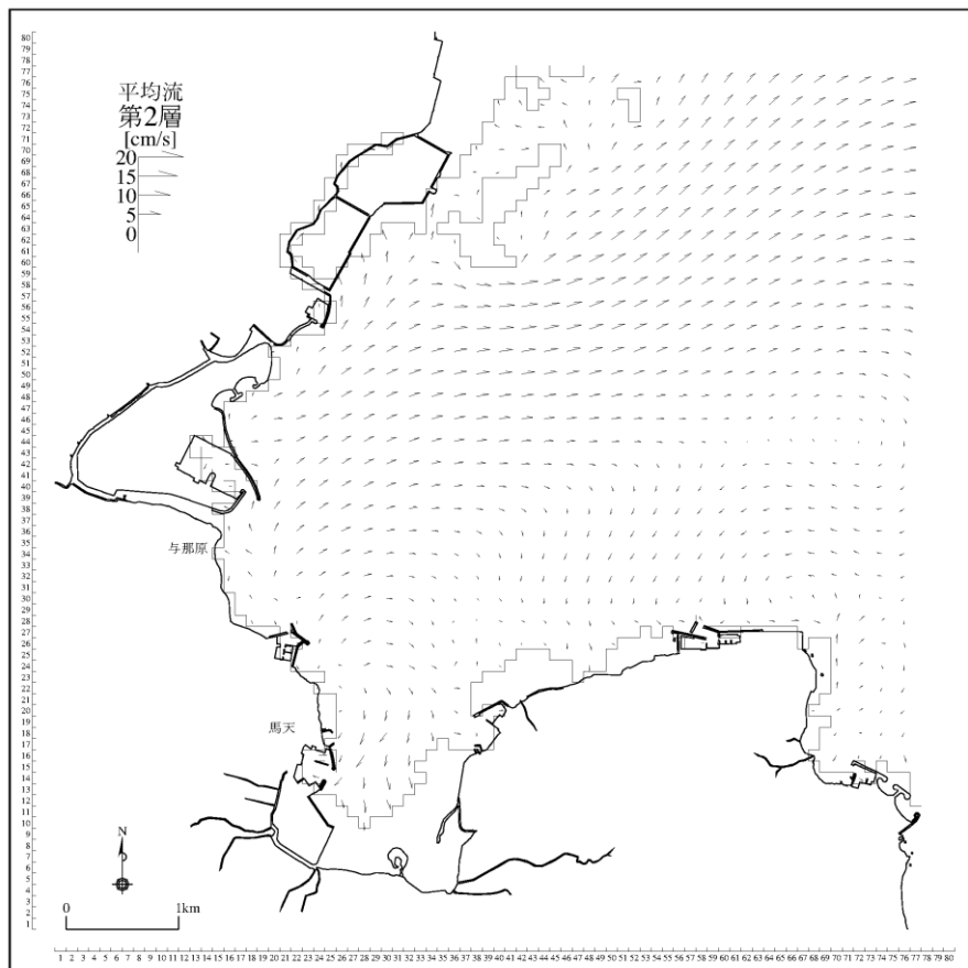
図 3-5-24(8) 将来潮流計算結果 (計画変更あり：夏季、恒流 (平均流) [第2層])
