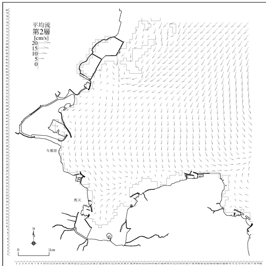
図 3-5-25(8) 将来潮流計算結果 (計画変更あり: 冬季、恒流 (平均流) [第2層])
