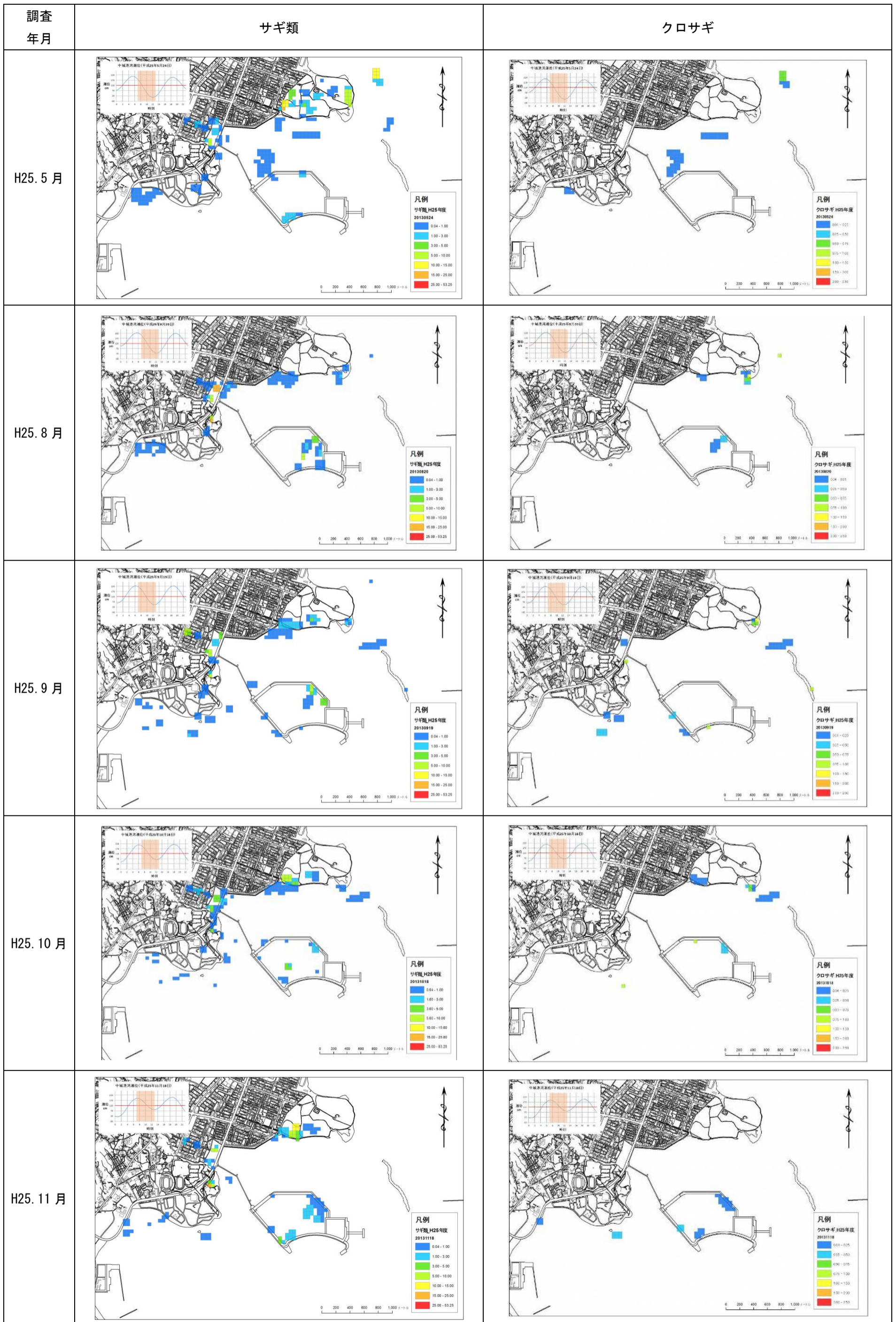
図1(2)-1 平成25年度のサギ類(左)及びクロサギ(右)の分布状況
