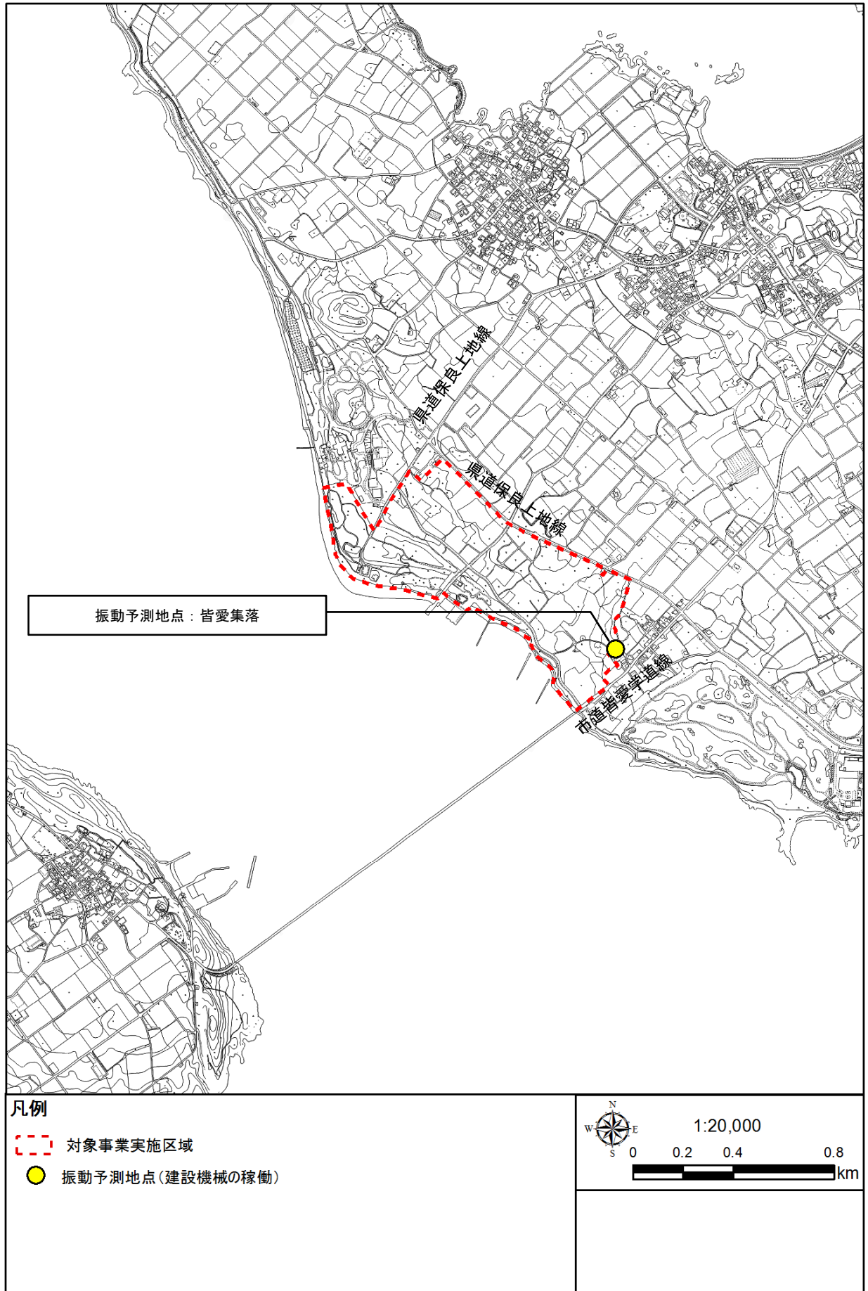
図 6.3.2-2 振動の予測地点（建設機械の稼働）
