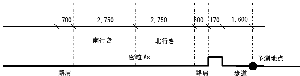
図 6.3.2-8(1) 予測地点の断面図 (市道皆愛学道線)
