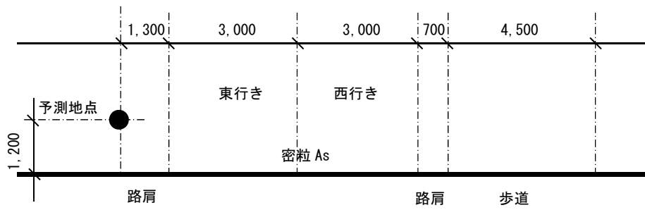
図 6.2.2-5(1) 予測地点の断面図 (県道保良上地線 (皆愛地区))
