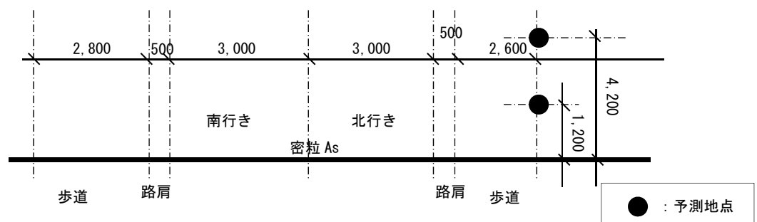
図 6.2.2-8(3) 予測地点の断面図 (県道保良上地線 (下地地区))
