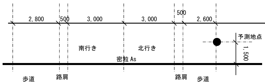
図 6.1.2-5 (2) 予測地点の断面図 (県道保良上地線 (下地地区))
