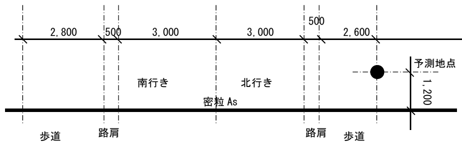
図 6.2.2-5(2) 予測地点の断面図 (県道保良上地線 (下地地区))
