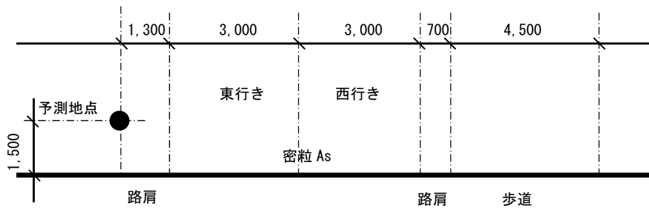
図 6.1.2-5 (1) 予測地点の断面図 (県道保良上地線 (皆愛地区))
