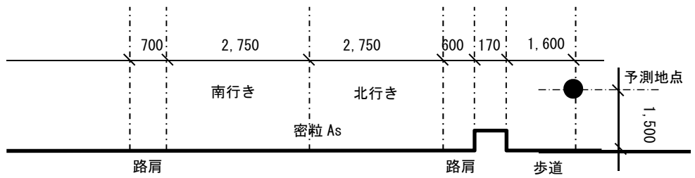
図 6.1.2-8(1) 予測地点の断面図 (市道皆愛学道線)
