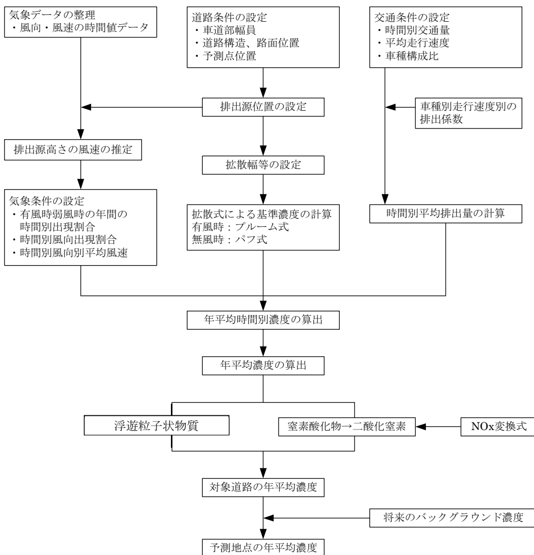
図 6.1.2-6 利用車両の走行に係る大気質の予測手順
