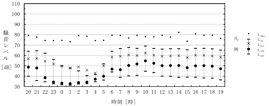
図 6.2.1-3(5) 道路交通騒音調査結果 (地点：県道保良上地線（下地地区）、春季の休日)
