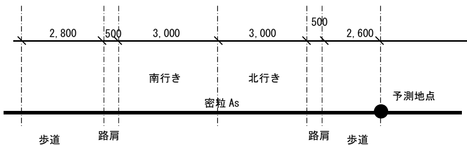
図 6.3.2-8(3) 予測地点の断面図 (県道保良上地線 (下地地区))
