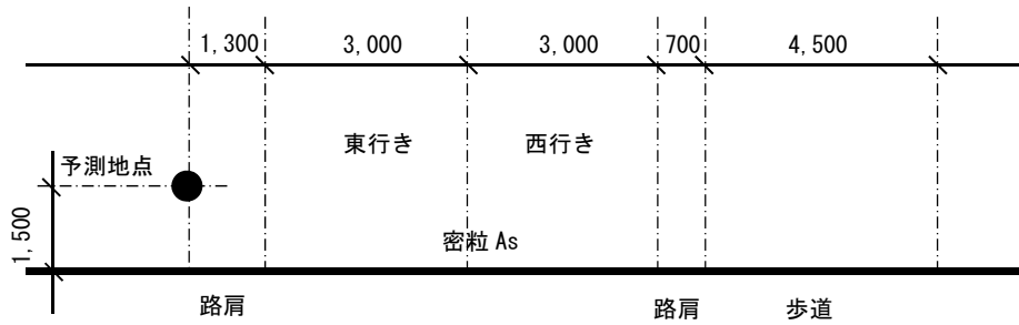
図 6.1.2-8(2) 予測地点の断面図 (県道保良上地線 (皆愛地区))
