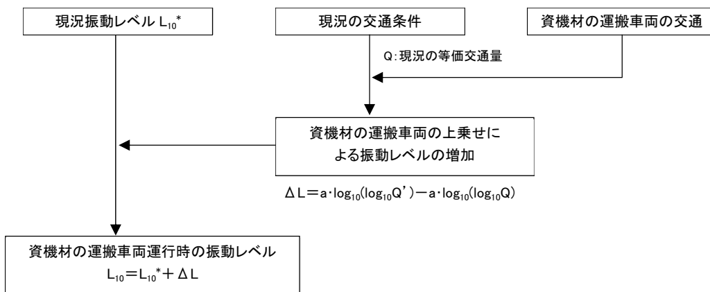
図 6.3.2-3 資機材の運搬車両の走行に係る振動の予測手順
