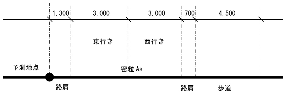
図 6.3.2-5(1) 予測地点の断面図 (県道保良上地線 (皆愛地区))
