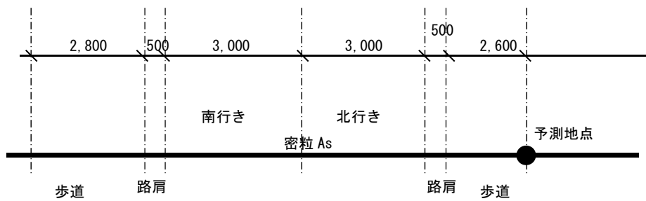
図 6.3.2-5(2) 予測地点の断面図 (県道保良上地線 (下地地区))
