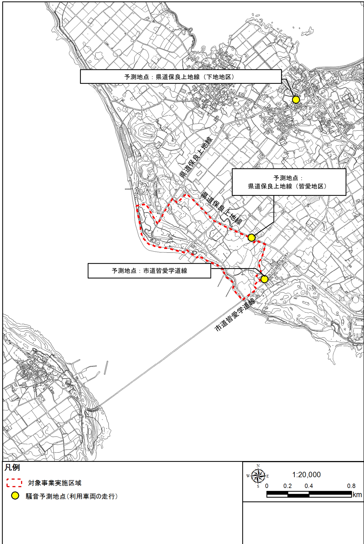
図 6.2.2-7 騒音の予測地点（利用車両の走行）
