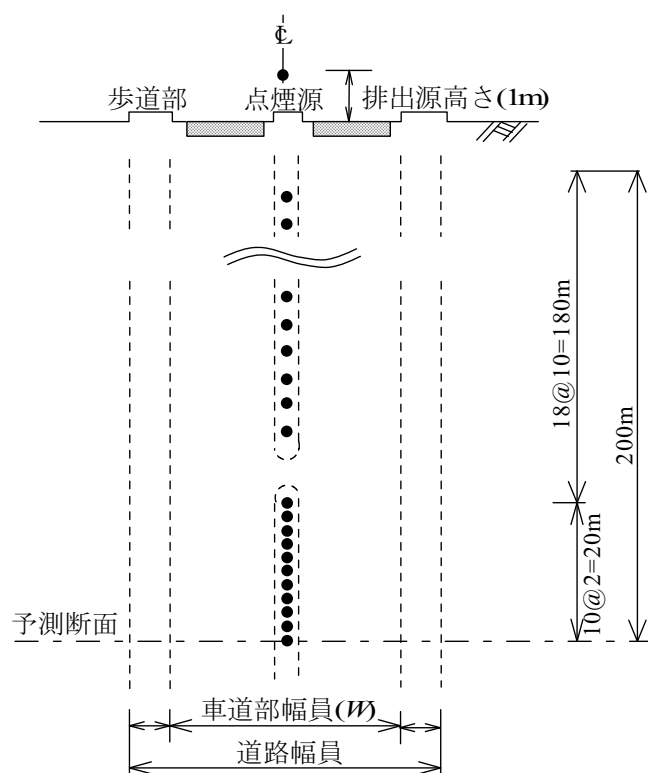
図 6.1.2-11 排出源の配置
