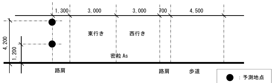
図 6.2.2-8(2) 予測地点の断面図 (県道保良上地線 (皆愛地区))
