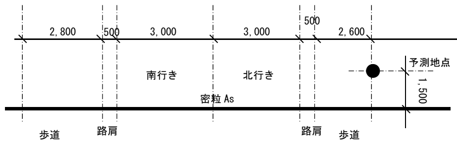
図 6.1.2-8(3) 予測地点の断面図 (県道保良上地線 (下地地区))
