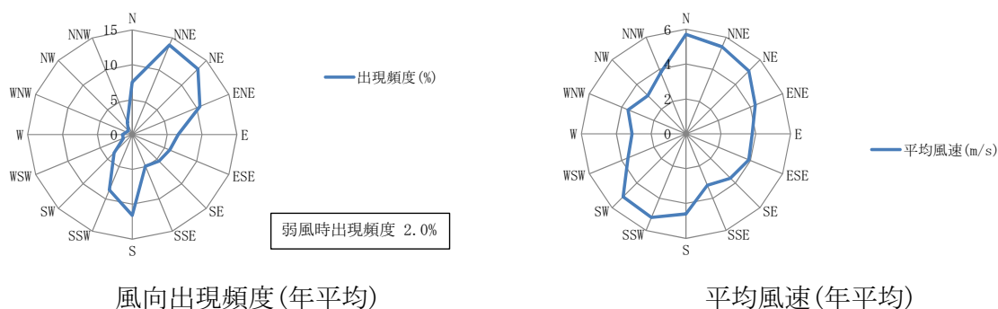
図 6.1.2-12 風配図及び風向別平均風速(年平均値)
