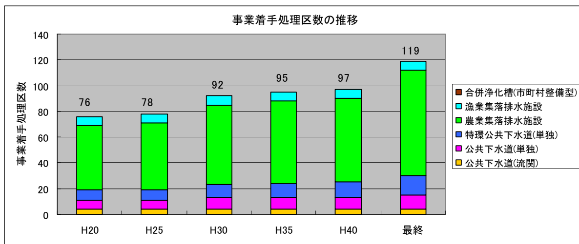
図 3-6 整備手法別事業着手処理区数の推移
