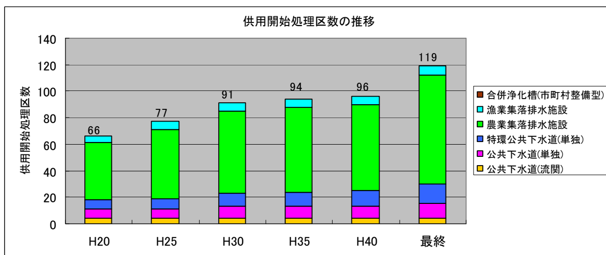
図 3-7 整備手法別供用開始処理区数の推移
