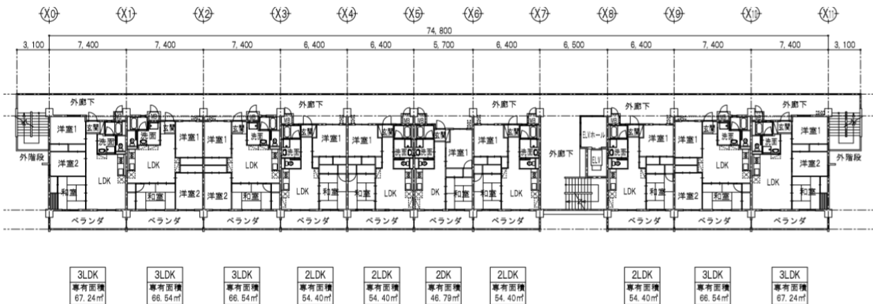
2~5階平面図 S=1:
