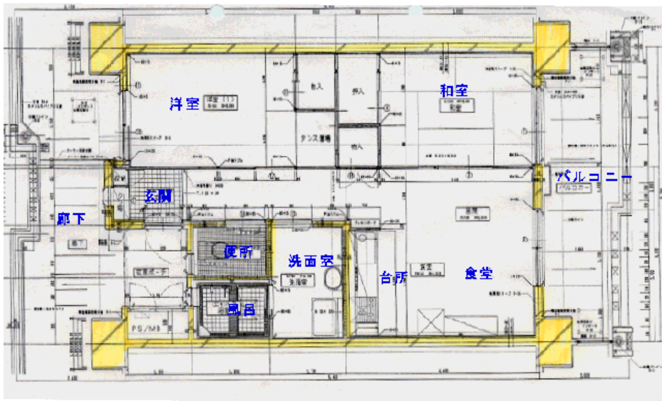
2LDK平面図
