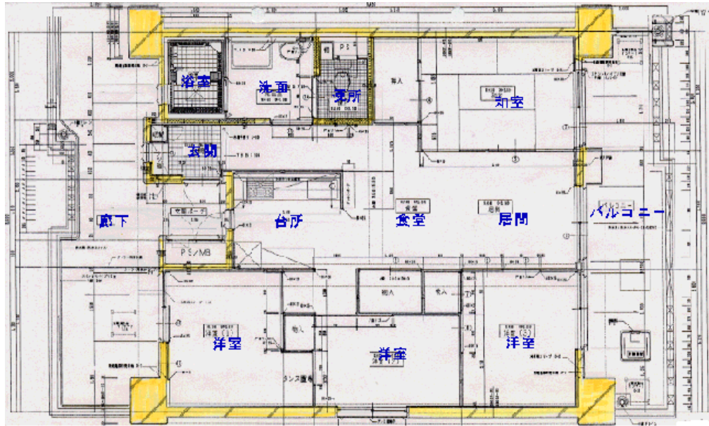
4LDK平面図
