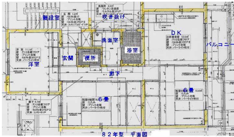
1～3棟 平面図
