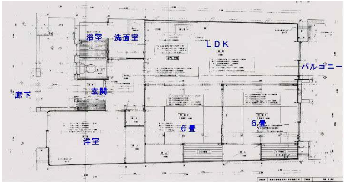
高層棟 平面図
