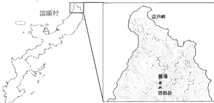
図-1 気象観測露場の設置位置図
