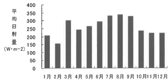
図-3 2010年 平均日射量 (W/m 2 )
