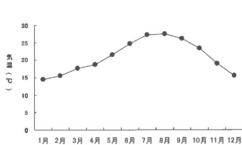
図-2 2010年 平均気温 (°C)
