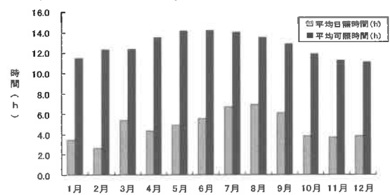
図-5 2010年月毎の平均日照時間 (h)
