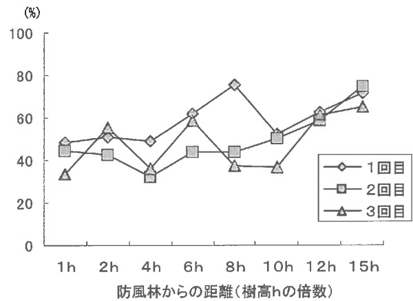
図-3 農研センター本所防風林②における減風率 (%) の計測結果
