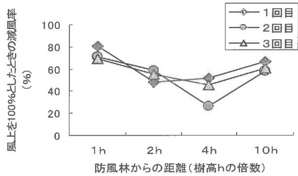
図-1 南大東島モクマウ防風林における減風率 (%)
