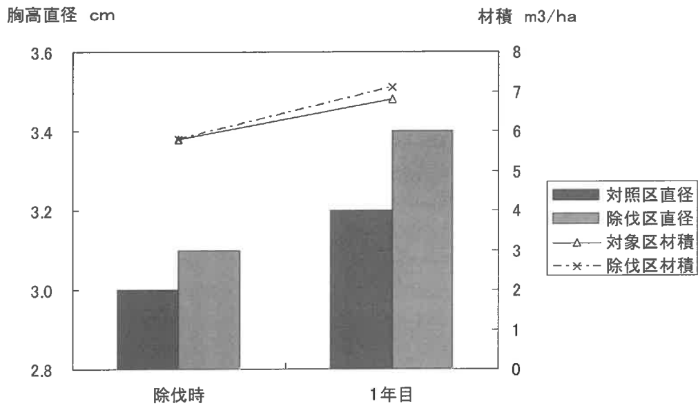
図一 1 胸高直径と材積（除伐試験）
