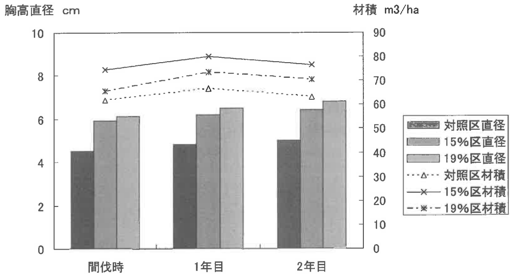
図一 2 胸高直径と材積（間伐試験）
