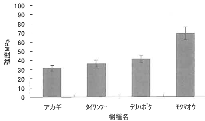
図-2 縦圧縮強度
