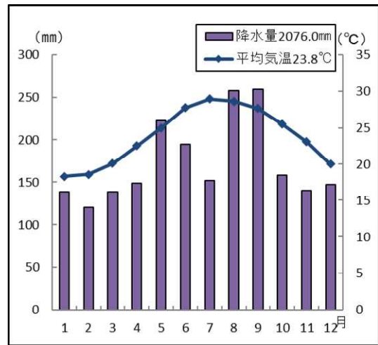
◎南大東島 (1991～2020年平均)
