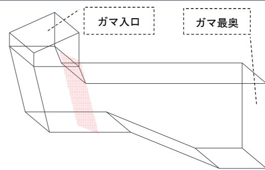
マヤーガンマ立面図 (C-4)
