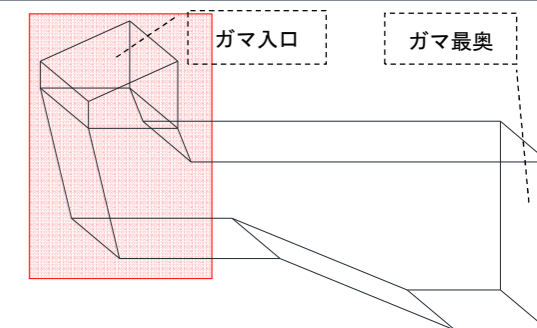
マヤーガンマ立面図 (C-5)
