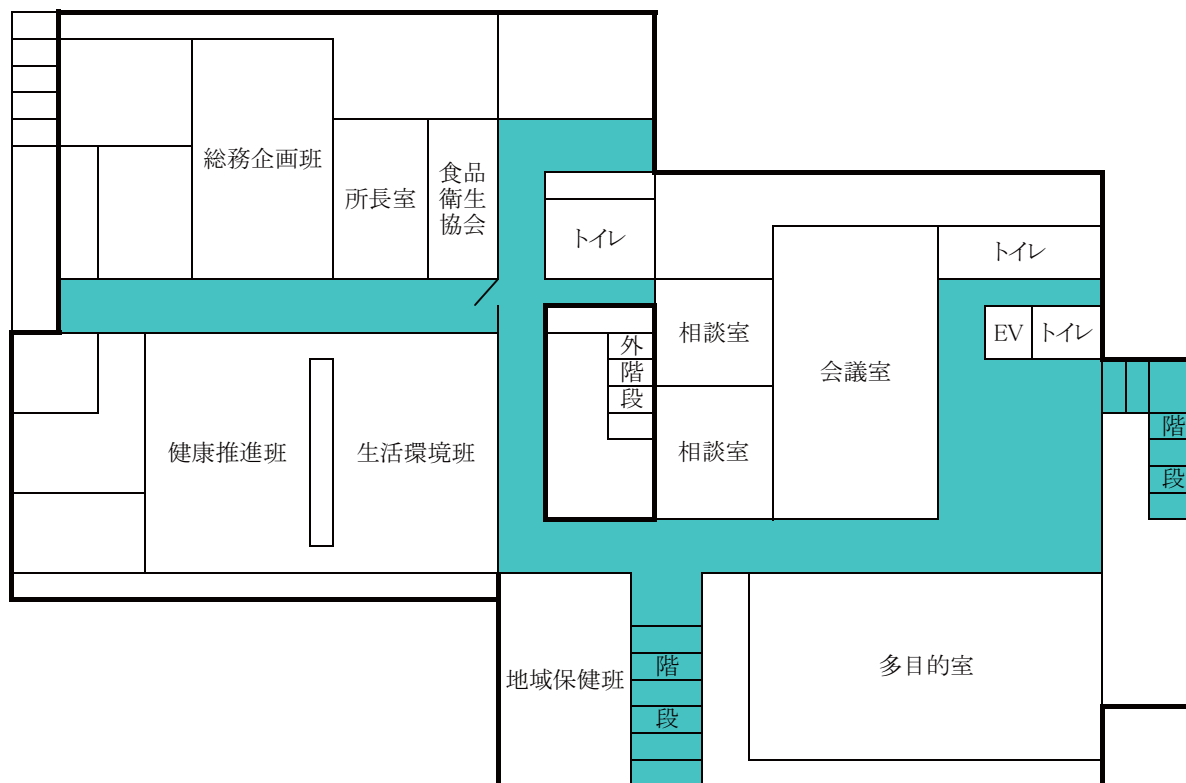
1階平面図
