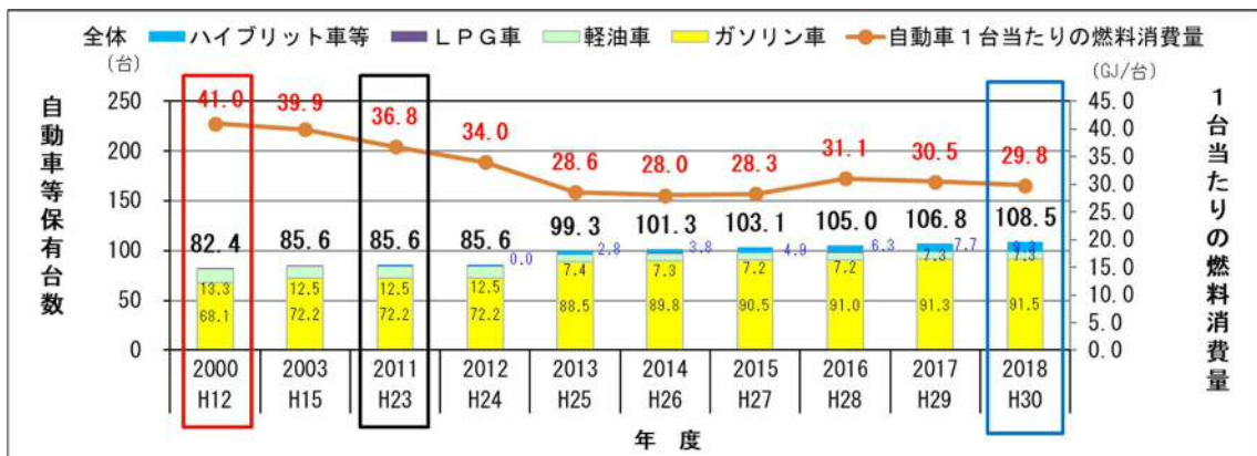
図3-4 自動車等保有台数と1台当たりの二酸化炭素排出量
