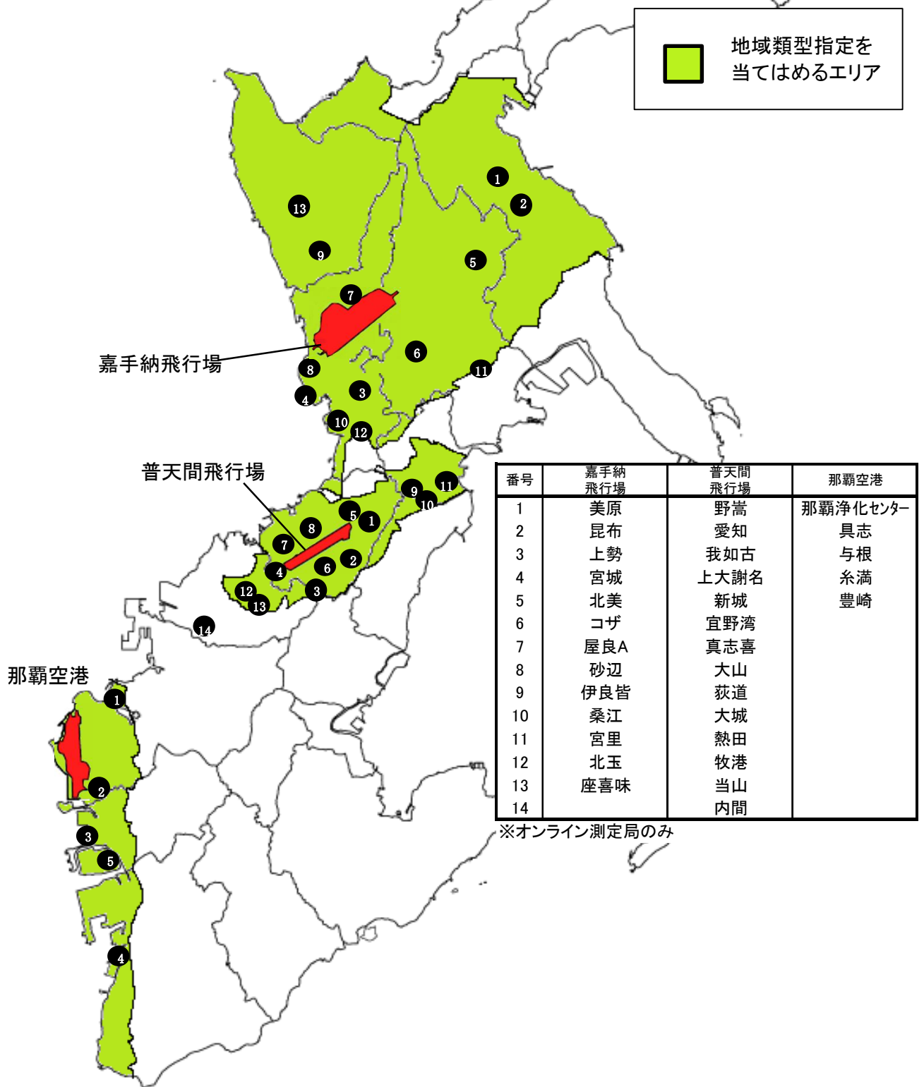
航空機騒音測定局配置図 (県とのオンライン測定局)
