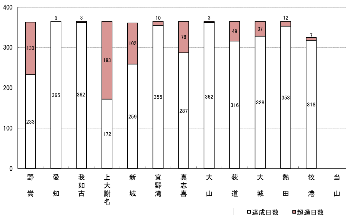
図 F 8 1日ごとのLdenが57dB又は62dBを超過した日数（普天間）
